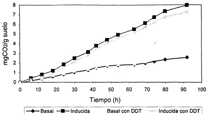
Figura 11. Producción de CO 2 como respuesta de actividad microbiana nativa en muestras de suelo B.
