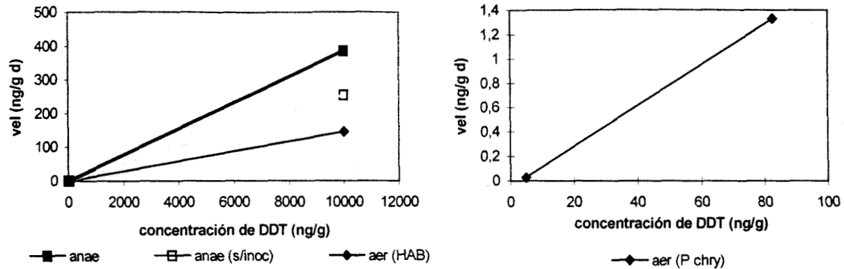
Figura 16. Gráficos de las velocidades de biodegradación contra la concentración inicial de DDT.
