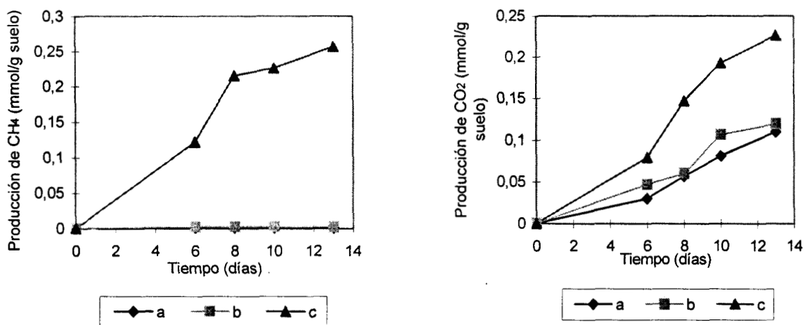
Figura 12. Producción de CH 4 y CO 2 en reactores anaerobios en presencia de DDT con: (a) suelo y agua, (b) suelo y nutrientes y (c) suelo, nutrientes y lodos.
