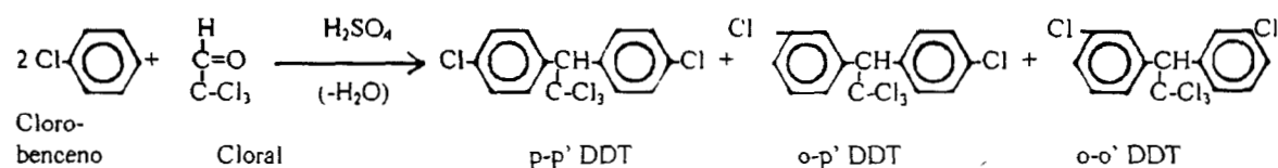
Figura 1. Reacciones durante la producción del DDT.
