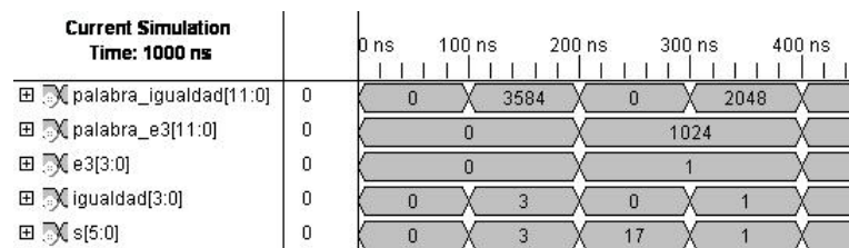
Figura 4.60: Simulación del componente Indicador de desplazamiento . La salida S indica la cantidad de desplazamientos que les deben ser realizados a los límites superior e inferior.
