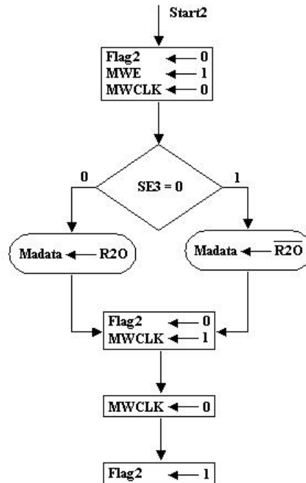
Figura 4.73: Diagrama de flujo de la maquina M0_R20.
