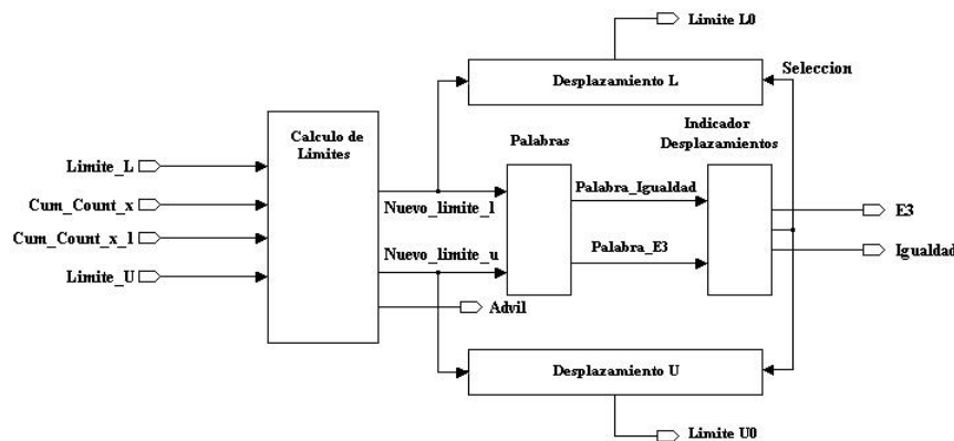
Figura 4.51: Diagrama interno del componente Cálculo del Intervalo, el cual calcula el intervalo correspondiente al símbolo recibido a la entrada y genera las señales de control necesarias para que la parte secuencial genere la etiqueta apropiada. Al ser descrito de forma combinacional, el tiempo de ejecución de este proceso sólo depende del tiempo de propagación del hardware.
