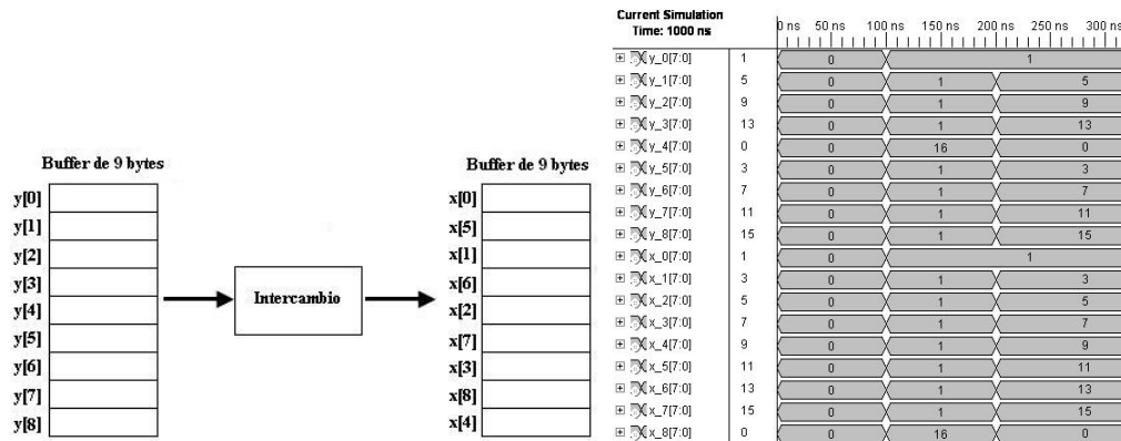
Figura 4.44: Simulación del funcionamiento del componente Intercambio. La información recibida a la entrada es reorganizada apropiadamente.
