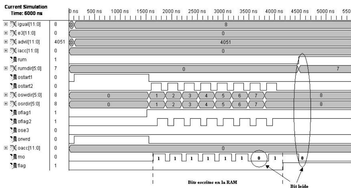
Figura 4.67: Bloque M0_R20, es una máquina de estados que realiza la copia.
