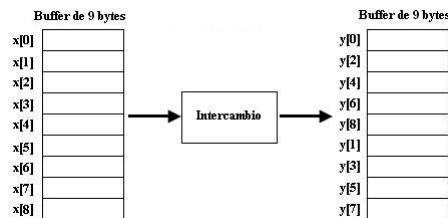
Figura 4.32: Esquema funcional del componente Intercambio. Reorganiza los datos almacenados en los arreglos fpb y fpa para que ahora sea el contenido de los renglones el que se encuentra en las posiciones consecutivas.
