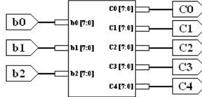
Figura 4.77: Componente Dispensor de nivel tres, efectúa la dispersión de manera completamente combinacional. Consta de tres entradas de ocho bits cada una ( b_0 ; b_1 ; b_2 ), por donde recibe los datos a dispersar, y cinco salidas ( C_0 ; C_1 ; C_2 ; C_3 ; C_4 ) de ocho bits cada una a través de las cuales entrega los datos ya dispersos.
