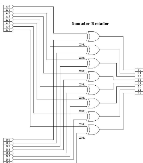
Figura 4.5: Diagrama del componente de nivel uno que efectúa las operaciones de suma y resta, que en el campo finito F_{2^8} son iguales. Este componente consiste en ocho compuertas XOR de dos entradas. Recibe en sus entradas A[7:0] y B[7:0] los datos en su representación polinomial, sobre los cuales efectúa la operación XOR bit a bit, generando un dato de ocho bits en la salida S[7:0] .
