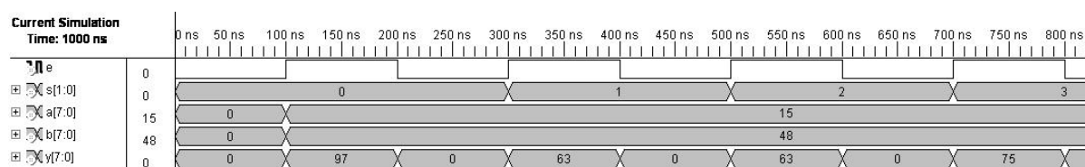
Figura 4.4: Simulación del componente de nivel tres Unidad Aritmética Lógica ALU . La combinación formada por los bits de las entradas S0 y S1 seleccionan el resultado de una de las cuatro operaciones realizadas por el componente (0=multiplicación, 1=suma, 2=resta y 3=división). Si la entrada E es puesta a cero, la salida será forzada a cero.
