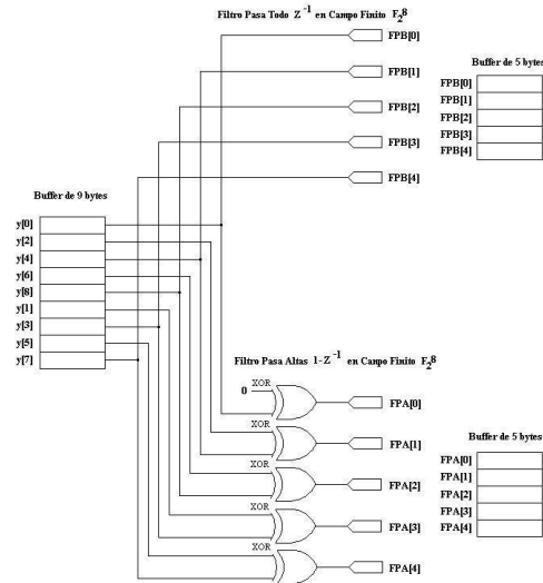
Figura 4.35: Diagrama de conexión de la etapa dos, en la cual se realiza el filtrado final de la imagen de tamaño 4 \times 4 .
