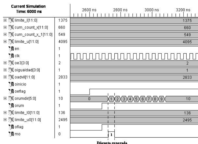
Figura 4.50: Simulación del compresor para el tercer caso, intervalo ya acotado pero que abarca tanto la porción inferior como la superior de la recta. La etiqueta generada es la correcta y se almacena el número correcto de condiciones E3 para ser consideradas en el procesamiento del siguiente elemento.
