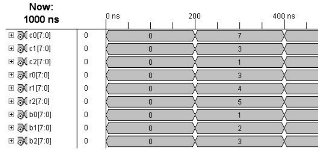
Figura 4.85: Simulación del componente Reconstructor de nivel cuatro. Los datos en las entradas c0 , c1 y c2 son los valores provenientes de los dispersos generados por los renglones 3, 4 y 5 de la matriz A , identificados en las entradas r0 , r1 y r2 . Los datos reconstruidos están en las salidas b0 , b1 y b2 .
