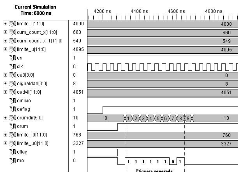
Figura 4.49: Simulación del segundo caso, límites muy cercanos a un extremo y entre ellos. La etiqueta resultante es larga, ya que ambos límites se parecen mucho entre ellos. Coincide con la etiqueta esperada.
