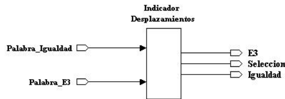
Figura 4.59: Componente Indicador de Desplazamiento , es un componente descrito combinatorialmente, basado en una tabla de verdad. Con la ayuda de dos vectores de entrada llamados: Palabra_Igualdad y Palabra_E3 , genera tres salidas llamadas: E3 , Igualdad y Selección , de las cuales las dos primeras pasaran a la segunda parte secuencial. La salida Selección indica cuantos desplazamientos a la izquierda de los límites se deben realizar.
