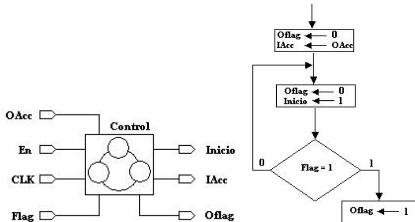
Figura 4.75: Componente de nivel dos que gestiona el adecuado funcionamiento entre las etapas secuencial y combinacional.
