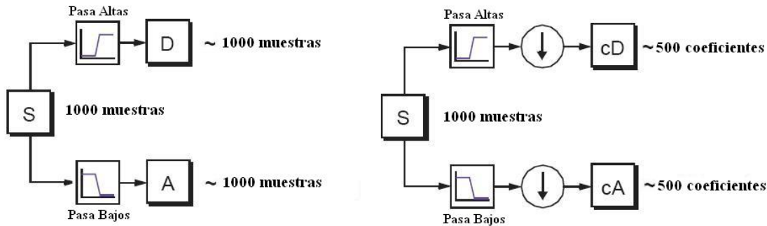
Figura 3.5: Al submuestrear las salidas de los filtros de aproximación y detalle se logra que el conjunto de A y D sea del mismo tamaño que la imagen original.
