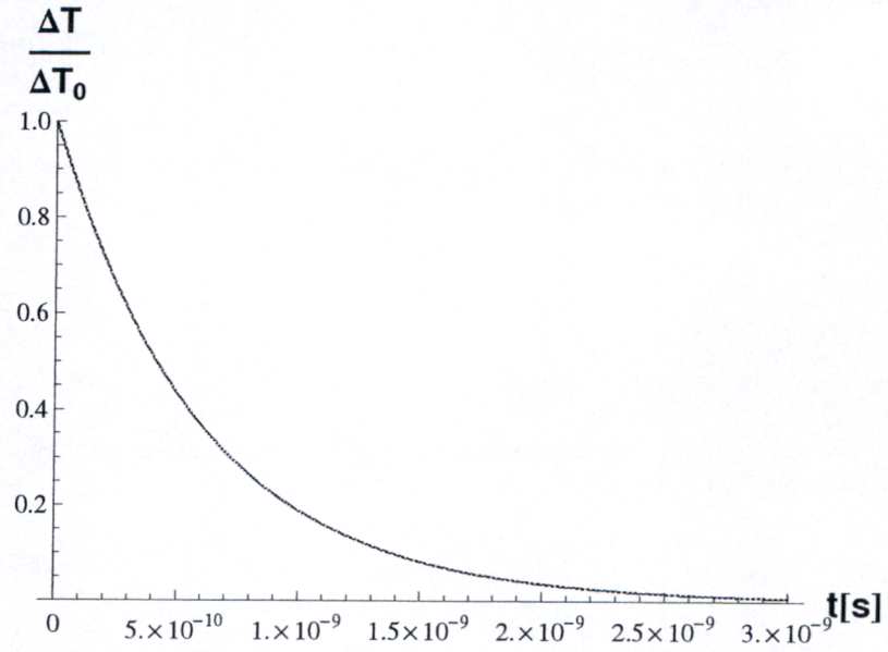
Figura 6.1: Decaimiento de la diferencia de temperaturas
