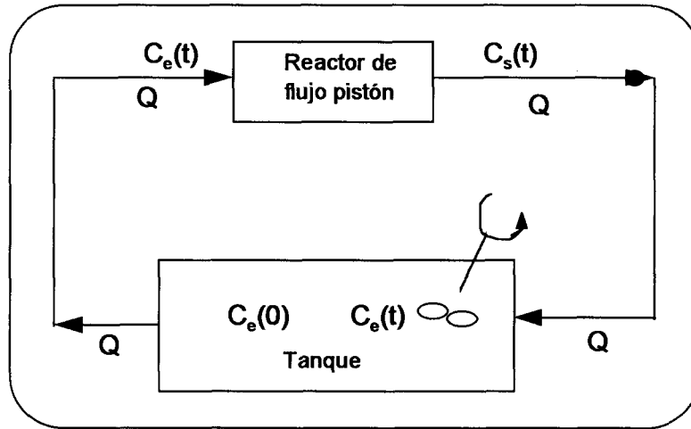
Figura AB.2 Arreglo de un reactor de flujo pistón en recirculación con un tanque con agitación.
