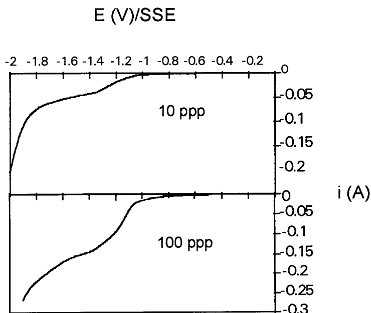
Figura 4.7 Curvas i - E para la reducción de Pb(II) 5 ppm en Na_2SO_4 0.5 M a pH 2, en CVR de 10 y 100 ppp. ( v=0.083 \text{ m/s} ). Velocidad de barrido de potencial de 5 mV/s.
