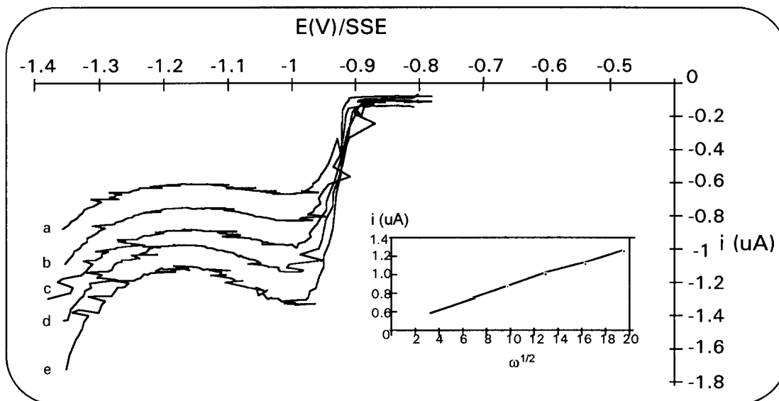
Figura 4.3 Curvas i - E para la reducción de Pb(II) 6 ppm en NaCl 0.5 M a pH 2, sin oxígeno, sobre un electrodo de disco rotatorio de carbón vítreo de A = 0.07 \text{ cm}^2 a diferentes velocidades de rotación a)400 r.p.m., b)900 r.p.m., c)1600 r.p.m., d)2500 r.p.m., y e)3600 r.p.m. Velocidad de barrido de potencial 5 mV/s. T = 25^\circ C . Se muestra también la gráfica i_L - \omega^{1/2} .
