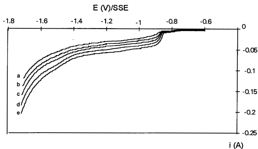
Figura 4.8 Curvas i - E para la reducción de Pb(II) 6 ppm en NaCl 0.5 M a pH 2 a diferentes velocidades lineales de flujo: a)0.05 m/s, b)0.083 m/s, c)0.125 m/s, d)0.166 m/s y e)0.25 m/s en un electrodo de CVR de 100 ppp. Velocidad de barrido de potencial de 5 mV/s. T = 25^{\circ}C .
