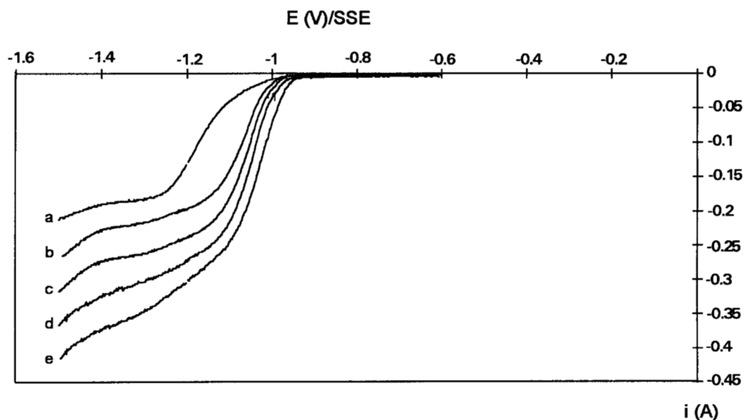
Figura 4.5 Curvas i - E para la reducción de Pb(II) 1 \cdot 10^{-3} M en NaNO 3 0.5 M a pH 2 a diferentes velocidades lineales de flujo: a)0.05 m/s, b)0.083 m/s, c)0.125 m/s, d)0.166 m/s y e)0.25 m/s en un electrodo de CVR de 10 ppp. Velocidad de barrido de potencial de 5 mV/s. T = 25°C.
