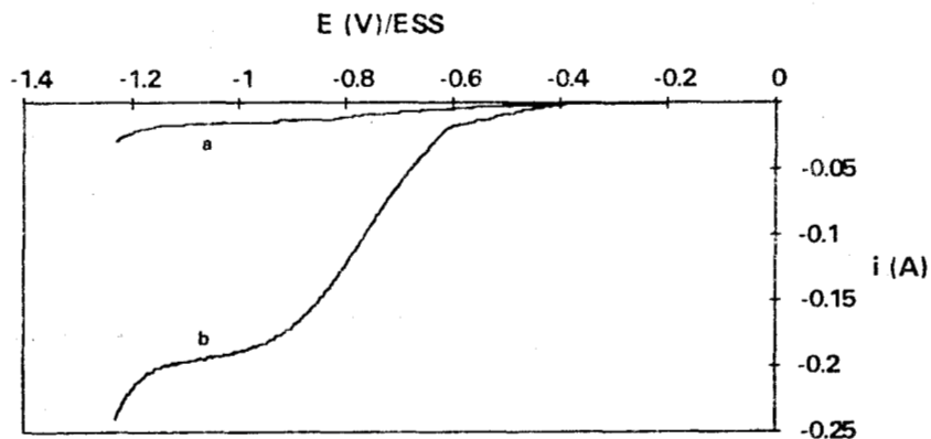
Figura 3.6 Curvas i - E para la reducción de \text{Cu(II)} 1 \cdot 10^{-3} \text{ M} en \text{Na}_2\text{SO}_4 0.5 \text{ M} a \text{pH } 2 en dos tipos de electrodos: a) Electrodo plano de carbón vítreo sólido con una área geométrica A = 25 \text{ cm}^2 y b) Electrodo de CVR de 10 ppp. A una velocidad lineal de flujo v de 0.083 \text{ m/s} . Velocidad de barrido de potencial 5 \text{ mV/s}
