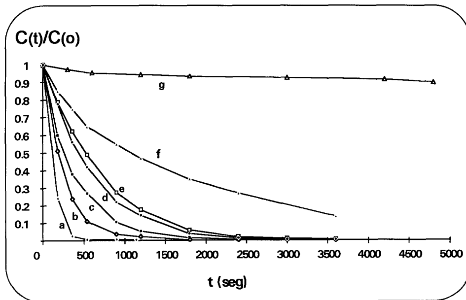
Figura 3.11 Decaimiento de la concentración del ion metálico \text{Cu(II)} 1 \cdot 10^{-3} \text{ M} en \text{Na}_2\text{SO}_4 0.5 \text{ M} pH 2 con respecto al tiempo durante la electrólisis, en diferentes electrodo: a)Fieltro, b)100 ppp, c)60 ppp, d)45 ppp, e)30 ppp, f)10 ppp y g)Electrodo plano. Potencial aplicado E = -1.14 \text{ V/SSE} . Velocidad lineal de flujo v = 0.083 \text{ m/s} . T = 25^\circ\text{C} y con purga de \text{N}_2 .
