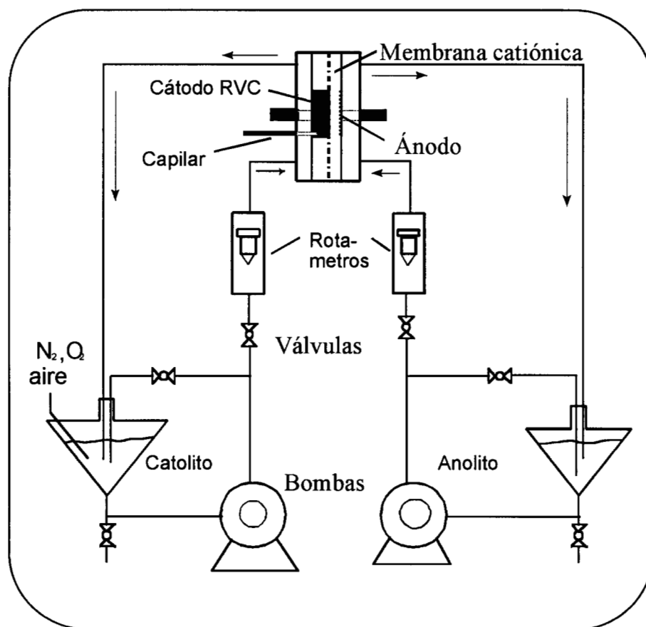
Figura 2.3 Diagrama esquemático del circuito hidráulico.
