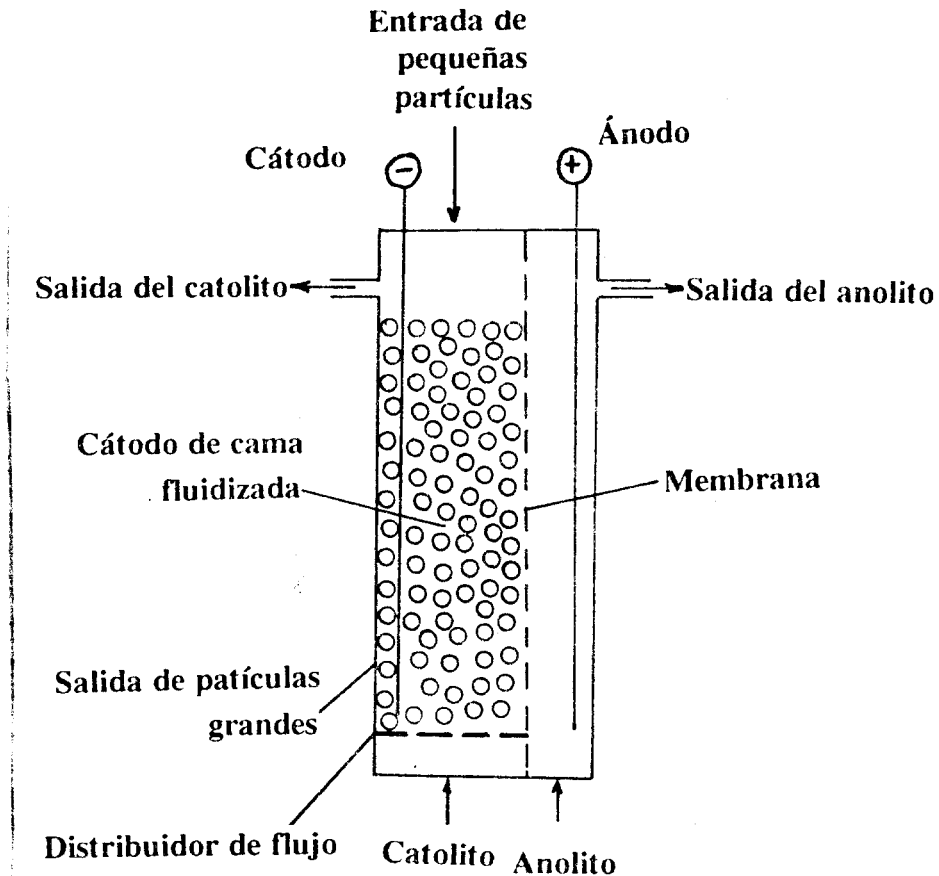
Figura 1.12 Diagrama esquemático de la celda de cama de lecho fluidizado.
