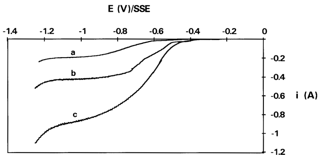
Figura 3.3 Curvas i - E para la reducción de Cu(II) 1 \times 10^{-3} M en Na_2SO_4 0.5 M a pH 2, a una velocidad de flujo \nu = 0.083 m/s para tres diferentes número de poros por pulgada: a)10 ppp, b)30 ppp y c)60 ppp. Velocidad de barrido de potencial 5 mV/s.
