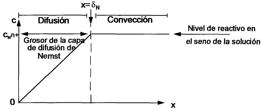
Figura 1.3 Perfil de la capa de difusión de Nernst en la interfase electrodo/electrolito en un sistema estacionario.
