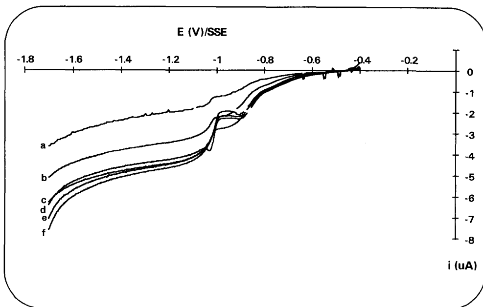
Figura 4.4 Curvas i - E para la reducción de Pb(II) 5 ppm en Na_2SO_4 0.5 M a pH 2, con oxígeno disuelto, sobre un electrodo de disco rotatorio de carbón vítreo de A = 0.07 \text{ cm}^2 a diferentes velocidades de rotación a)100 r.p.m., b)400 r.p.m., c)900 r.p.m., d)1600 r.p.m., e)2500 r.p.m., y f)3600 r.p.m. Velocidad de barrido de potencial 5 mV/s. T = 25^\circ\text{C} .
