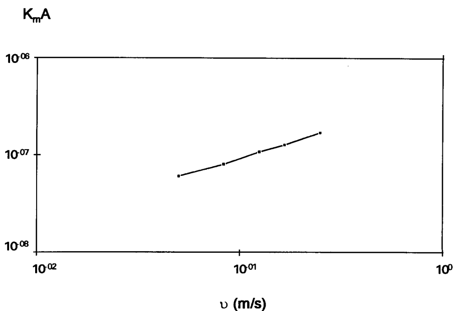
Figura 3.7 Gráfica log-log del producto K_m A como una función de la velocidad lineal de flujo v para un electrodo plano de carbón vítreo sólido de área A = 25 \text{ cm}^2 , para el sistema \text{Cu(II)} 1 \cdot 10^{-3} \text{ M} en \text{Na}_2\text{SO}_4 0.5 \text{ M} a pH 2. La corriente límite i_L fue leída a un potencial E de -1.14 \text{ V/SSE} de la figura 3.5.
