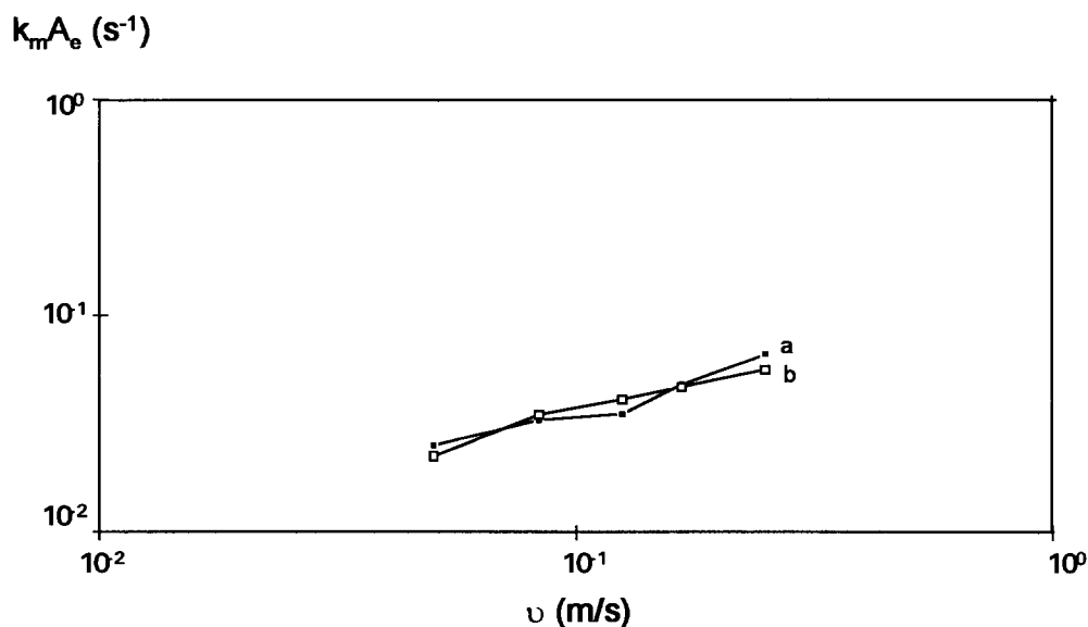
Figura 4.6 Gráfica log-log del producto K_m A_e como una función de la velocidad lineal de flujo para un electrodo de 10 ppp. a) Pb(II) 1 \cdot 10^{-3} \text{ M} en \text{NaNO}_3 0.5 M a pH 2 y b) Cu(II) 1 \cdot 10^{-3} \text{ M} en \text{Na}_2\text{SO}_4 0.5 M a pH 2.
