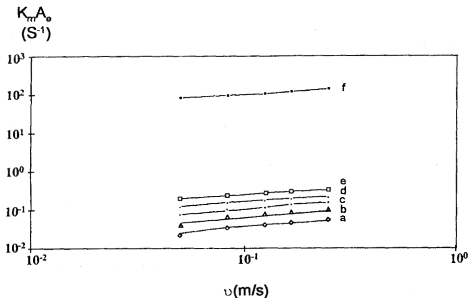
Figura 3.9 Gráfica log-log del producto K_m A_e como una función de la velocidad lineal de flujo v para un electrodo de f) Fieltro de grafito comparado con electrodos de CVR de diferente número de poros por pulgada: a)10 ppp, b)30 ppp, c)45 ppp, d)60 ppp, y e)100 ppp. Para el sistema Cu(II) 1 \cdot 10^{-3} M en Na_2SO_4 0.5 M a pH 2. La corriente límite i_L para el fieltro fue leída a un potencial E de -1.14 V/SSE de la figura 3.8.
