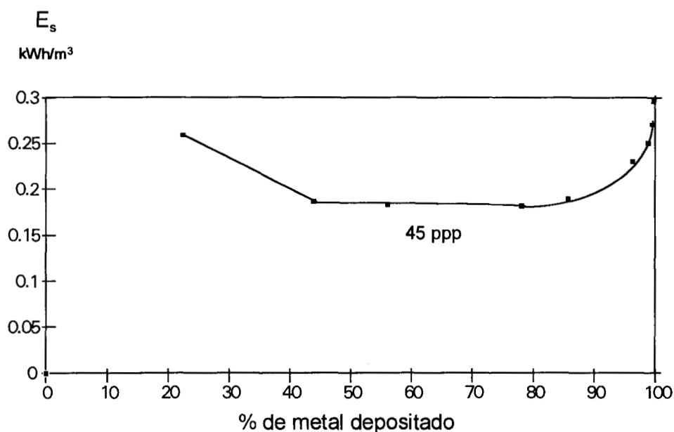
Figura 3.13 Variación de la energía de consumo E_s con respecto al % de metal depositado en un electrodo de 45 ppm durante la electrólisis.
