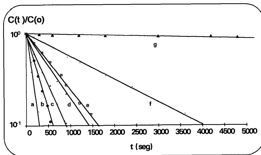
Figura 3.12 Logaritmo del decaimiento de la concentración de \text{Cu(II)} 1 \cdot 10^{-3} \text{ M} en \text{Na}_2\text{SO}_4 0.5 \text{ M} pH 2 con respecto al tiempo durante la electrólisis, en diferentes electrodo: a)Fieltro, b)100 ppp, c)60 ppp, d)45 ppp, e)30 ppp, f)10 ppp y g)Electrodo plano. Potencial aplicado E = -1.14 \text{ V/SSE} . Velocidad lineal de flujo v = 0.083 \text{ m/s} . T = 25^\circ\text{C} y con purga de \text{N}_2 .
