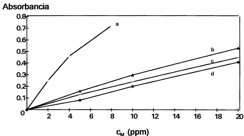
Figura AD.1 Curvas de calibración para absorción atómica. a)Cu(II) 1 mM en \text{Na}_2\text{SO}_4 0.5 M pH 2, b)Pb(II) 1 mM en \text{NaNO}_3 0.5 M pH 2, c)Pb(II) 6 ppm en \text{NaCl} 0.5 M pH 2, d)Pb(II) 5 ppm en \text{Na}_2\text{SO}_4 0.5 M pH 2.
