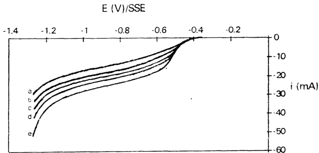
Figura 3.5 Curvas i - E obtenidas para la reducción de \text{Cu(II)} 1 \cdot 10^{-3} \text{ M} en \text{Na}_2\text{SO}_4 0.5 \text{ M} a \text{pH } 2 con un electrodo plano de carbón vítreo sólido de área geométrica A = 25 \text{ cm}^2 a diferentes velocidades lineales de flujo v : a) 0.05 \text{ m/s} , b) 0.083 \text{ m/s} , c) 0.125 \text{ m/s} , d) 0.166 \text{ m/s} y e) 0.25 \text{ m/s} . Velocidad de barrido de potencial de 5 \text{ mV/s} . T = 25^\circ\text{C} .
