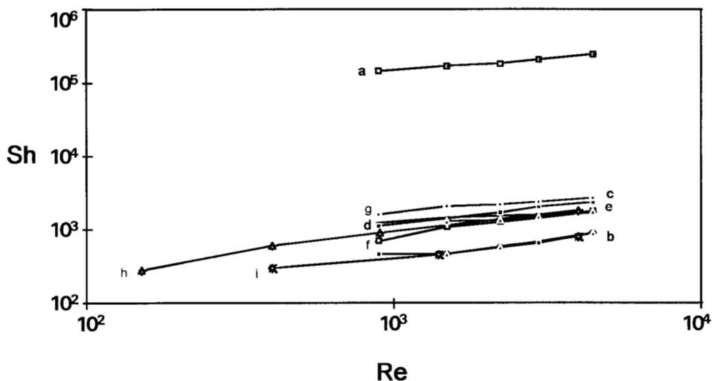
Figura 3.10 Correlación Sh-Re obtenida en el reactor estudiado para diferentes formas geométricas de electrodos: a)Filtro, b)Electrodo plano de carbón vítreo sólido, c)CVR de 60 ppp, d)CVR de 100 ppp, e)CVR de 45 ppp, f)CVR de 30 ppp, g)CVR de 10 ppp h)Correlación obtenida por Pletcher [10] para un electrodo de CVR y i)Correlación obtenida por Pletcher [10] para un electrodo plano.
