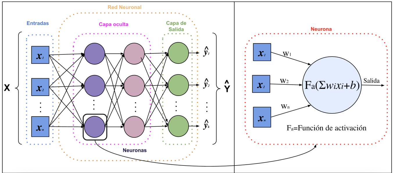
Figura 3.2: Esquema de una red neuronal con sus capas de entrada, ocultas y de salida. Así como la estructura de una neurona; donde a la suma ponderada de todas las entradas se le aplica la función de activación ( f_a ).
