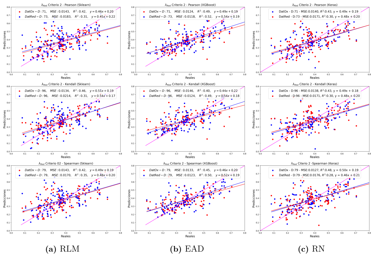
Figura 11.7: Gráficas de dispersión para los tres modelos de ajuste que predicen la energía de reorganización \lambda_{Red} considerando el Criterio 2 y las distintas formulaciones de correlación.
