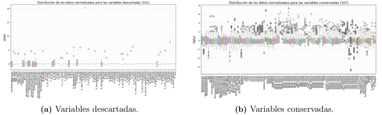
Figura 5.3: Gráficas de cajas para las variables normalizadas de la familia de la Bpy, provenientes del DatRed. La Figura (a) contiene a las variables descartadas por su baja variabilidad mientras que la Figura (b) muestra las variables conservadas por su mayor variabilidad.
