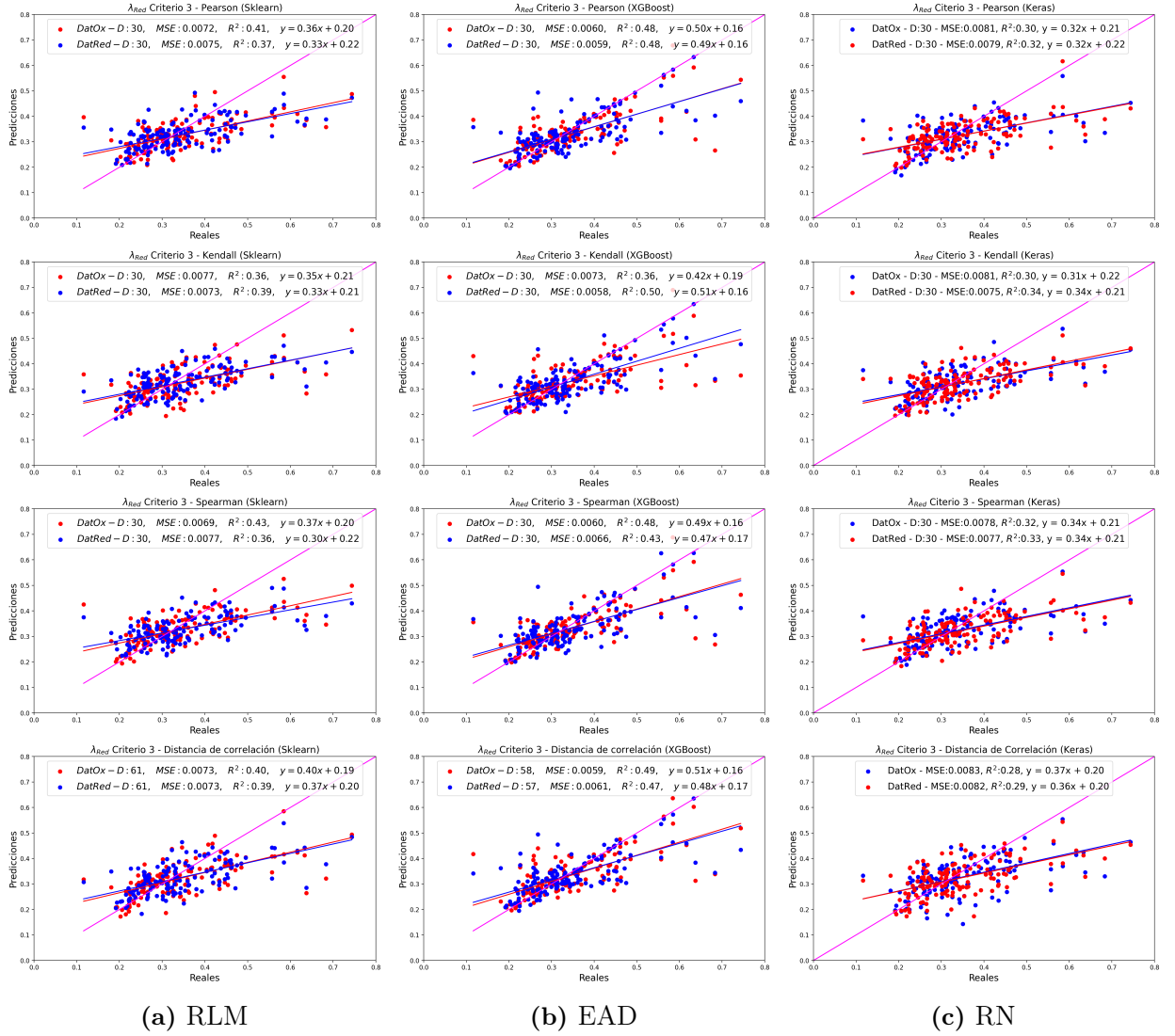
Figura 11.20: Gráficas de dispersión para los tres modelos de ajuste que predicen la energía de reorganización \lambda_{Red} considerando el Criterio 3 y las distintas formulaciones de correlación.
