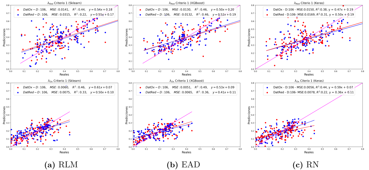
Figura 11.5: Gráficas de dispersión (Bz) para los tres modelos de ajuste que predicen la energía de reorganización \lambda_{\text{Red}} y \lambda_{\text{Ox}} respectivamente considerando el Criterio 1.
