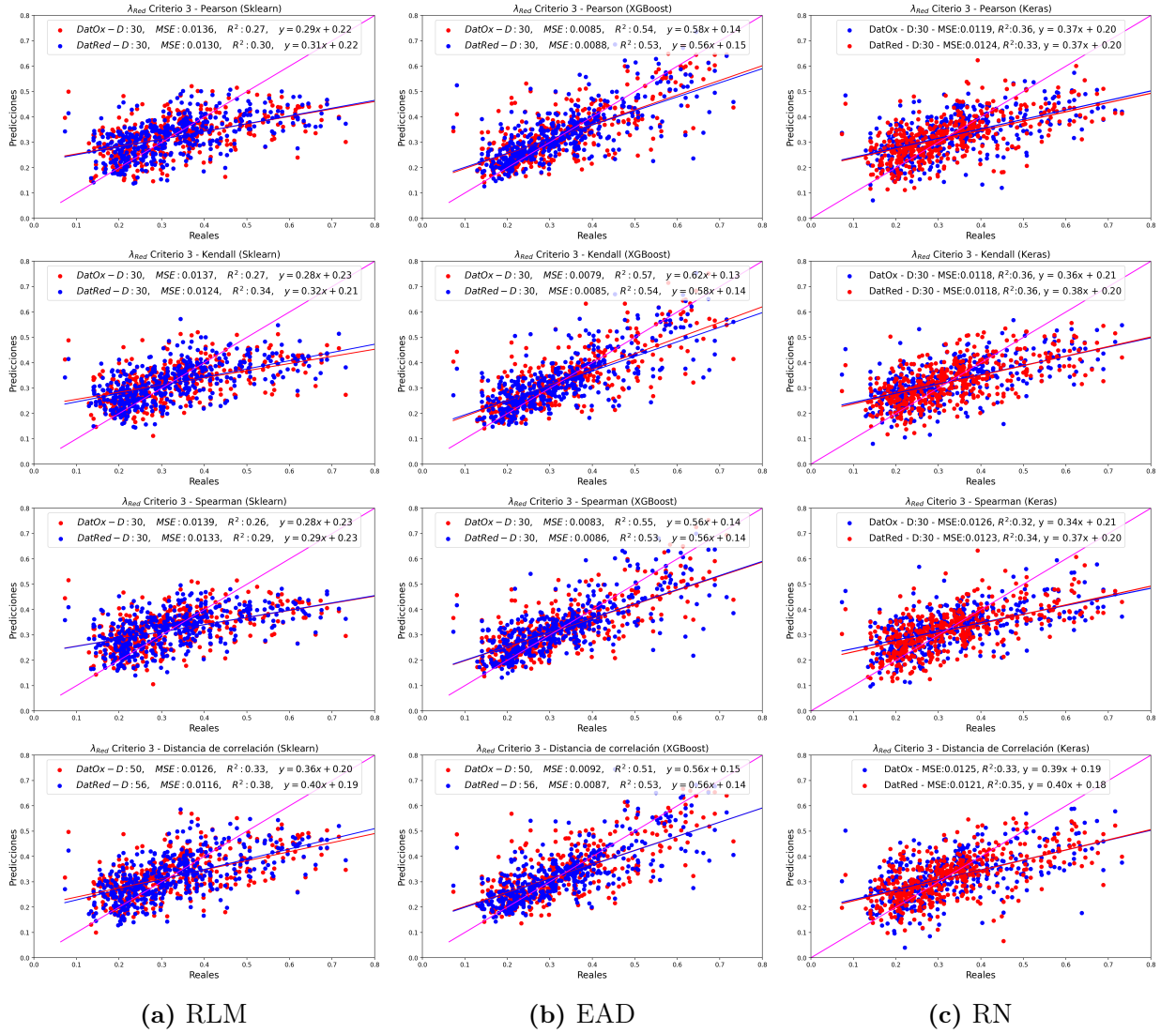
Figura 8.5: Gráficas de dispersión para el conjunto de todas la familias con los tres modelos de regresión que predicen la energía de reorganización \lambda_{\text{Red}} considerando el Criterio 3 y las distintas formulaciones de correlación.
