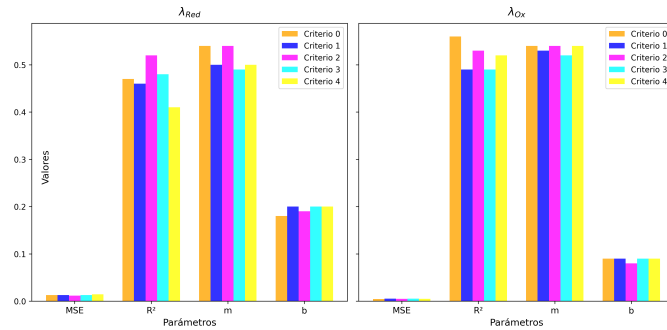
Figura 6.5: Evolución de las métricas de rendimiento en función de los criterios para ambas energía de reorganización. Los datos corresponden a los mejores modelos presentados en las Tablas: Criterio 0: 6.1; Criterio 1: 6.2; Criterio 2: 6.3 y 6.4; Criterio 3: 6.5 y 6.6; Criterio 4: 6.9.
