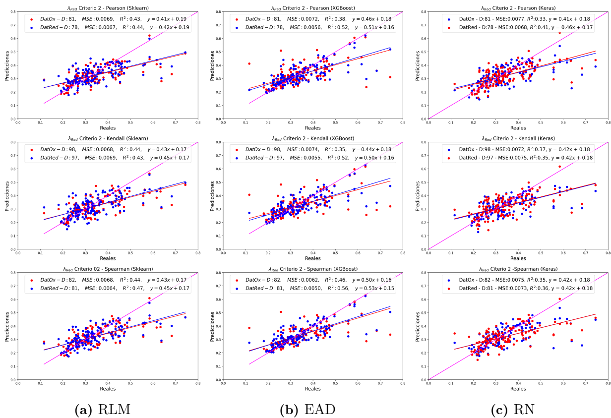
Figura 11.18: Gráficas de dispersión para los tres modelos de ajuste que predicen la energía de reorganización \lambda_{Red} considerando el Criterio 2 y las distintas formulaciones de correlación.
