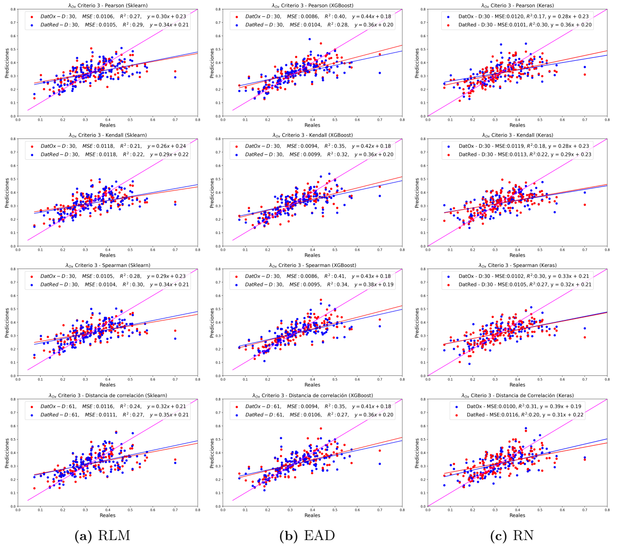
Figura 11.21: Gráficas de dispersión (de la familia de las MV's) para los tres modelos de ajuste que predicen la energía de reorganización \lambda_{Ox} considerando el Criterio 3 y las distintas formulaciones de correlación.
