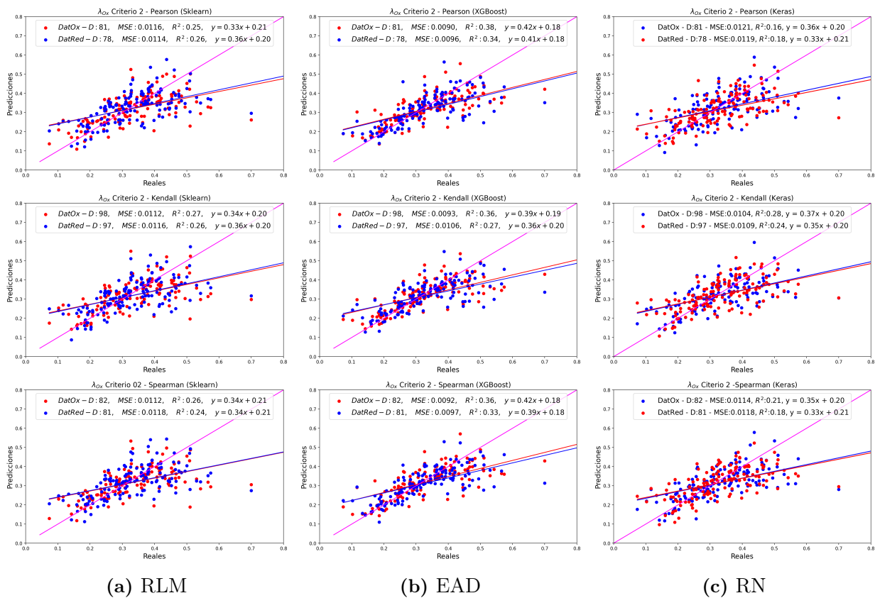
Figura 11.19: Gráficas de dispersión para los tres modelos de ajuste que predicen la energía de reorganización \lambda_{Ox} considerando el Criterio 2 y las distintas formulaciones de correlación.
