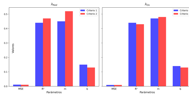
Figura 5.10: Comparación de los parámetros de rendimiento entre el criterio 1 y el criterio 2. Los datos corresponden a los mejores modelos presentados en las Tablas: Criterio 1: 5.2; Criterio 2: 5.3.
