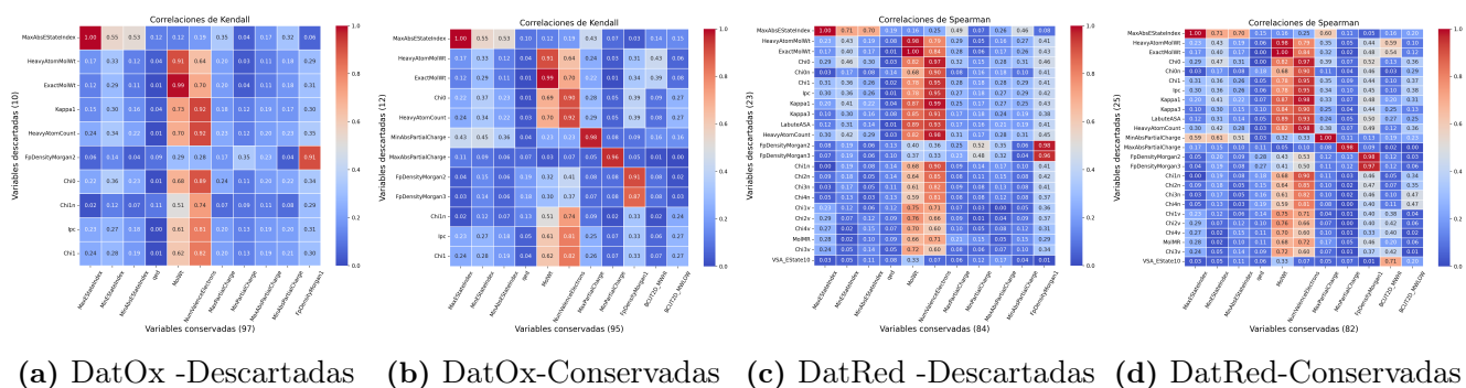
Figura 5.7: Matrices de correlación de Kendall en primer renglón y Spearman en el segundo para distintos métodos y base de datos. El código de colores indica que entre mas intenso sea el color rojo hay un correlación alta entre ambas variables. Mientras que la intensidad del color tienda hacia el azul hay una baja correlación
