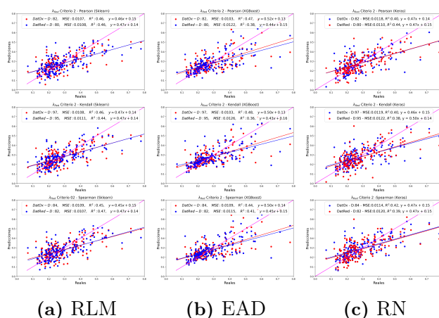
Figura 5.8: Gráficas de dispersión para los tres modelos de ajuste que predicen la energía de reorganización \lambda_{Red} considerando el Criterio 2 y las distintas formulaciones de correlación. Pearson (primer renglón), Kendall (segundo renglón) y Spearman (tercer renglón).
