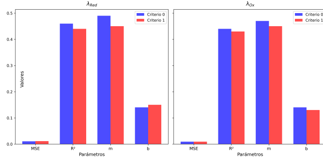
Figura 5.5: Comparación de las métricas de rendimientos entre el criterio 0 y el 1. Las métricas son los valores en azul de las Tablas 5.1 (criterio 0) y 5.2 (criterio 1).
