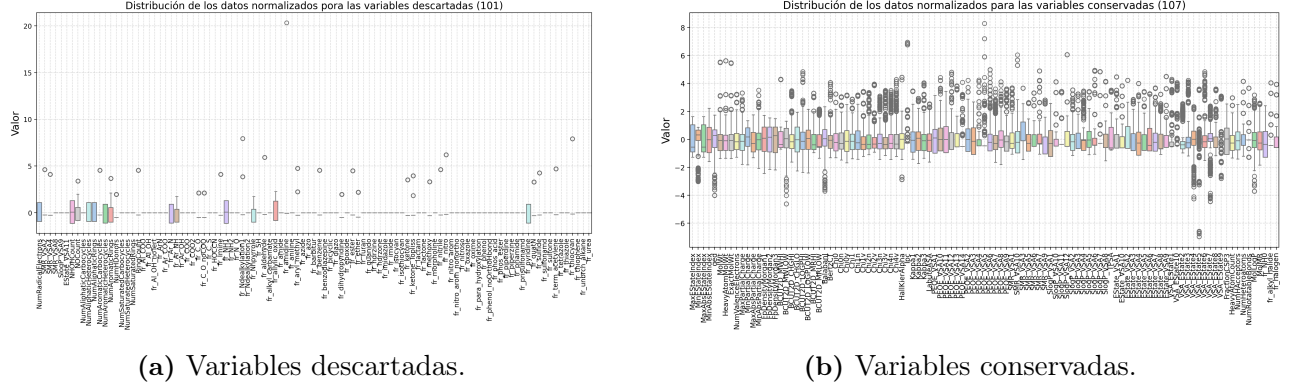
Figura 5.2: Gráficas de cajas para las variables normalizadas de la familia de la Bpy, provenientes del DatOx. En la que describen la varianza de los datos. La Figura (a) contiene a las variables descartadas por su baja variabilidad mientras que la Figura (b) muestra las variables conservadas por su mayor variabilidad.
