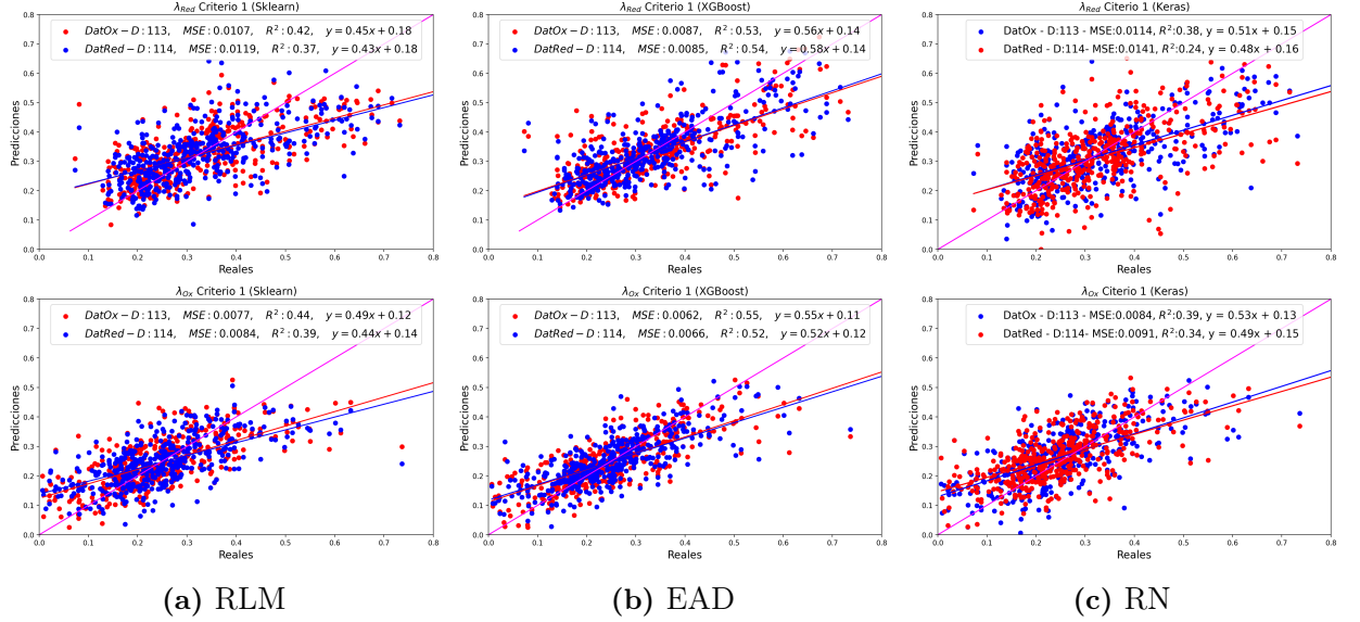
Figura 8.2: Gráficas de dispersión (para el conjunto de todas las familias) para los tres modelos de ajuste que predicen la energía de reorganización \lambda_{\text{Red}} y \lambda_{\text{Ox}} respectivamente considerando el Criterio 1.
