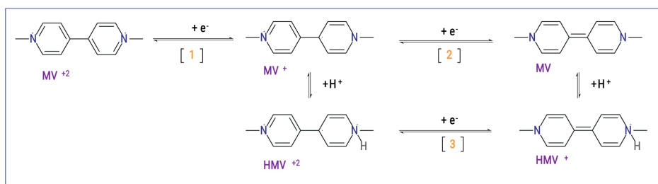
Figura 4.4: Esquema reaccional de los procesos monoelectrónicos para el MV.
