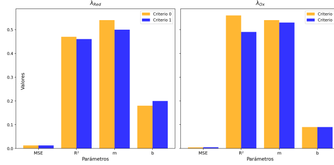
Figura 6.2: Evolución de las métricas de rendimiento en función de los criterios para ambas energía de reorganización. Los datos corresponden a los mejores modelos presentados en las Tablas: Criterio 0: 6.1; Criterio 1: 6.2.
