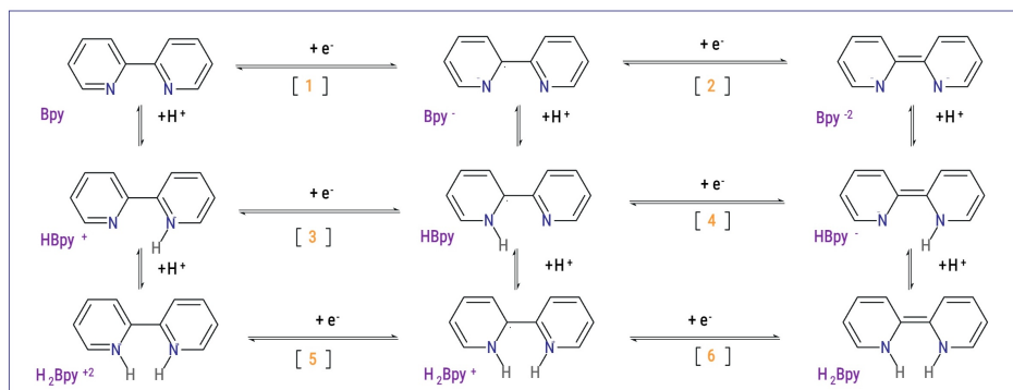
Figura 4.5: Esquema reaccional de los procesos monoelectrónicos para la Bpy.
