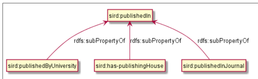
Figura 4.17: Jerarquía de propiedades para vincular a una organización con un recurso digital.
