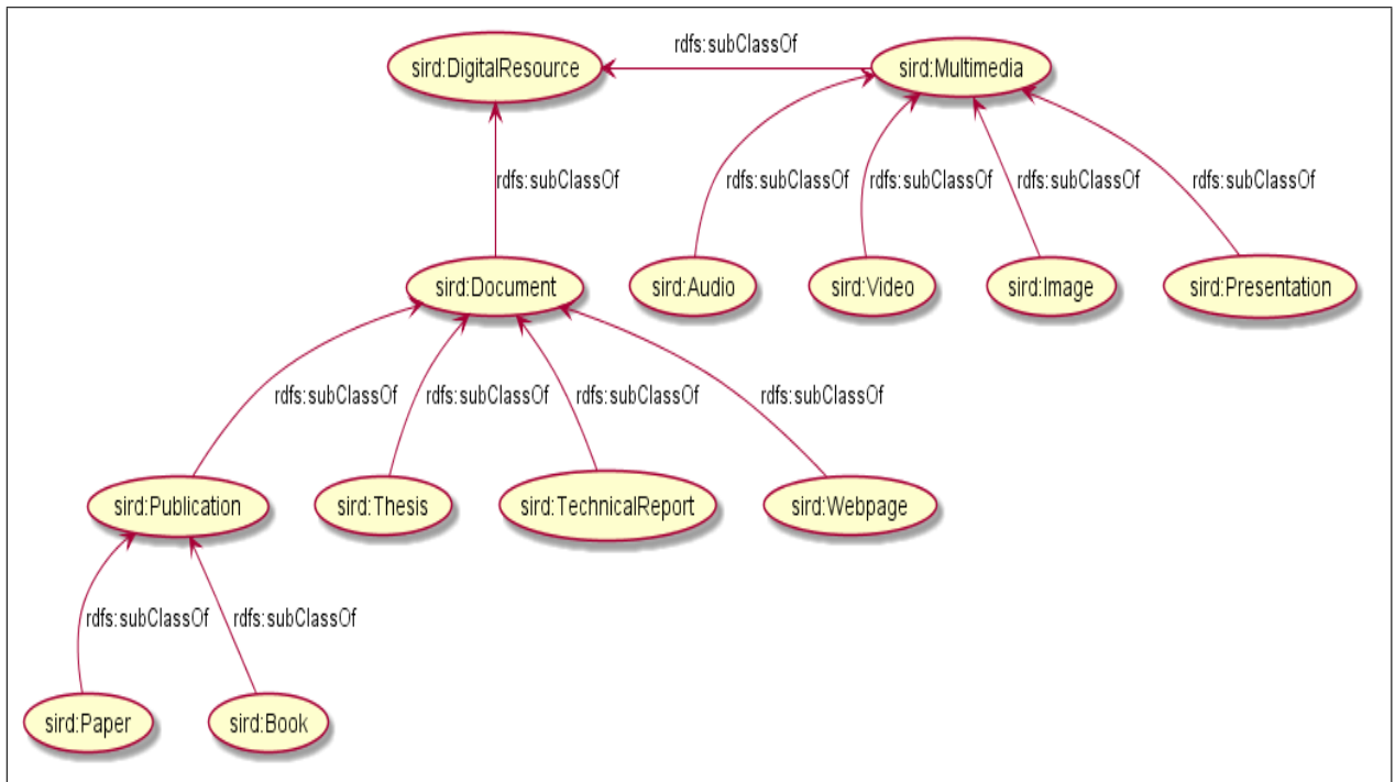
Figura 4.10: Jerarquía de clases para los recursos digitales
