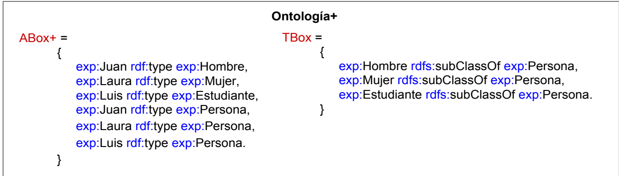
Figura 2.7: Ontología con tripletas que han sido inferidas mediante un razonador.
