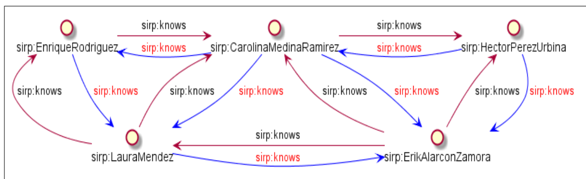
Figura 4.26: Ejemplo de inferencia a partir de la propiedad conoce-a como propiedad simétrica.
