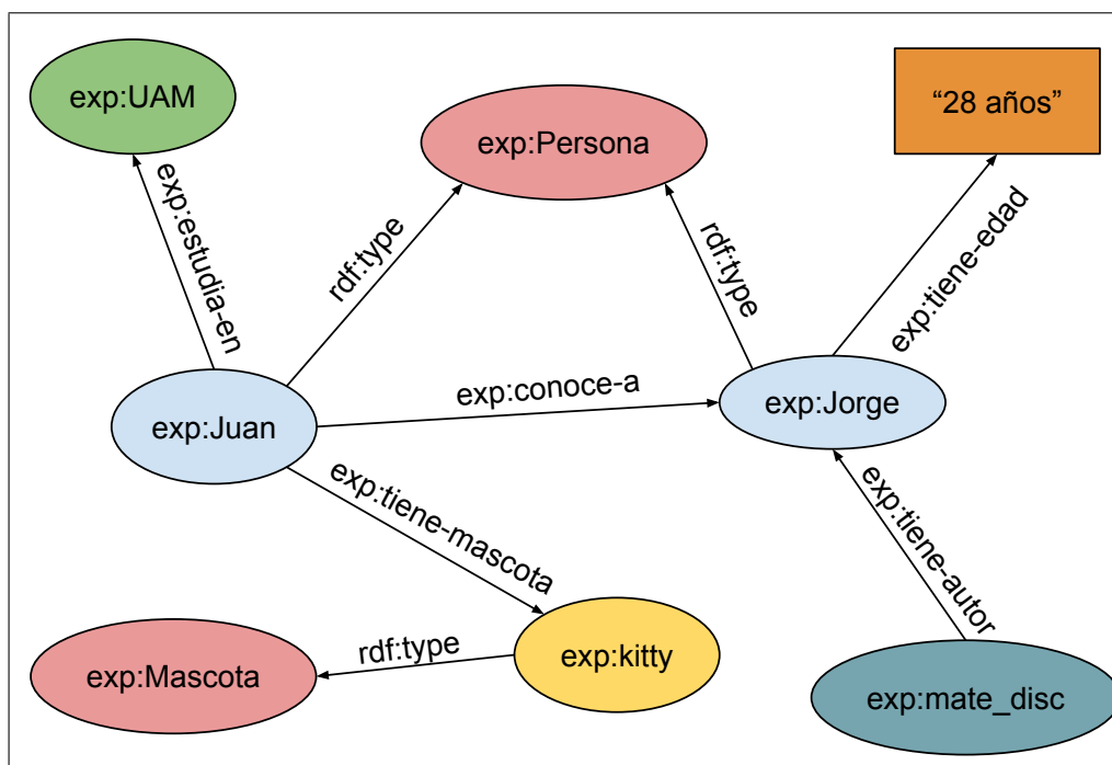
Figura 2.2: Ejemplo de un grafo RDF o grafo de conocimientos.
