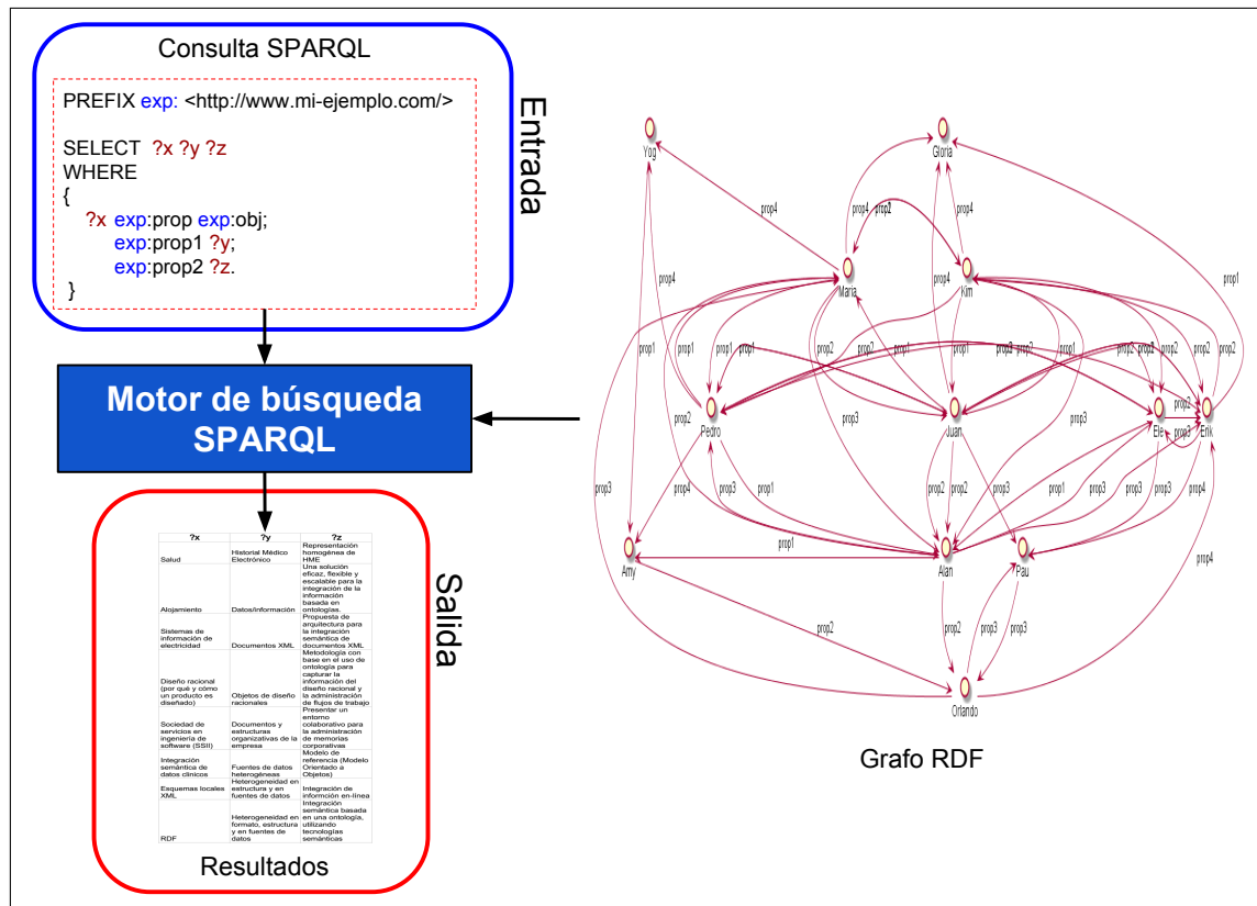
Figura 4.32: Proceso básico de consulta de información para un motor de búsqueda SPARQL.
