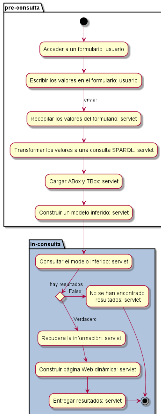
Figura 5.1: Flujo básico de la interacción de un usuario con un servlet.
