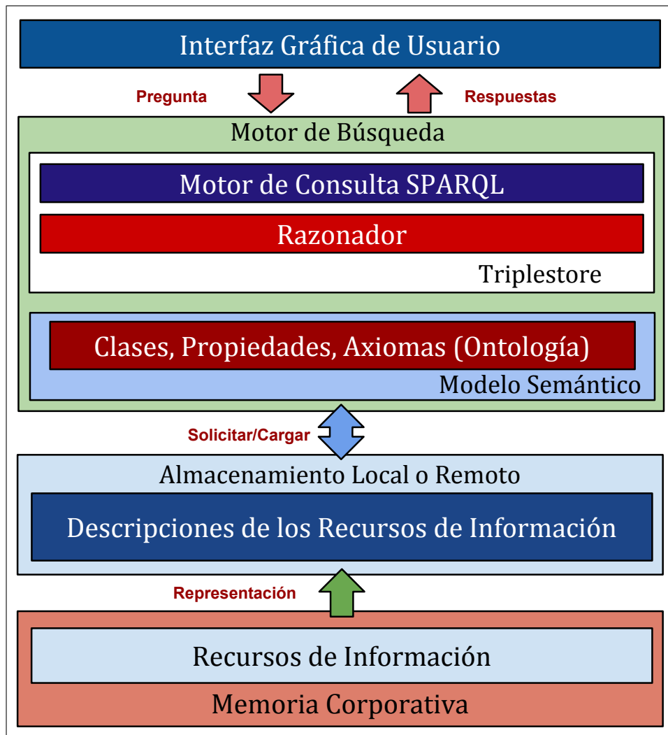
Figura 4.1: Arquitectura general para la integración semántica de recursos de información en una memoria corporativa.
