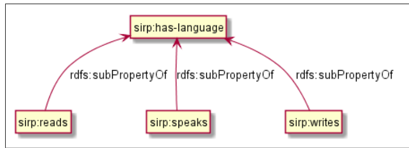
Figura 4.12: Jerarquía de propiedades para las habilidades lingüísticas.
