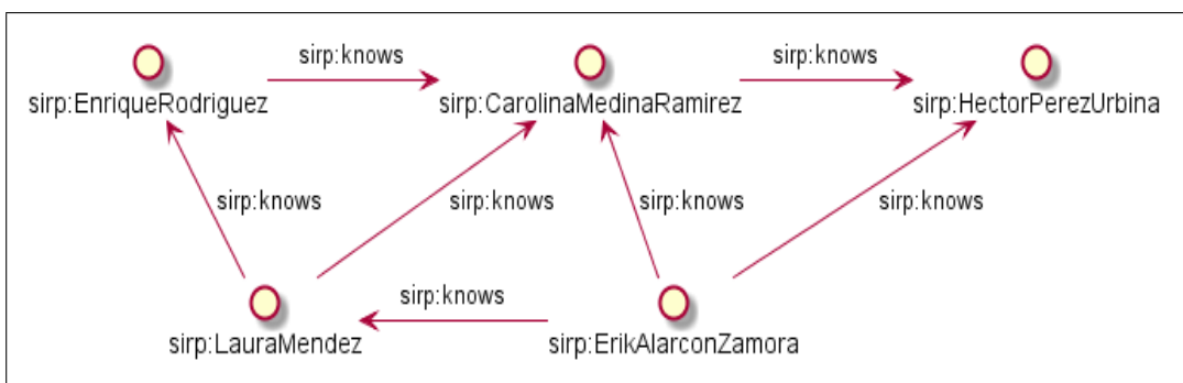
Figura 4.25: Subgrafo RDF de las relaciones conoce-a entre personas del área de redes y telecomunicaciones.
