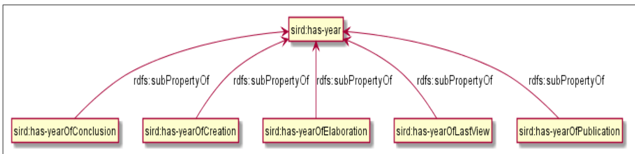
Figura 4.16: Jerarquía de propiedades para indicar el año de un recurso digital.
