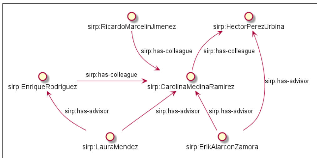
Figura 4.19: Tripletas RDF que describen las relaciones profesionales entre personas del área de redes y telecomunicaciones.
