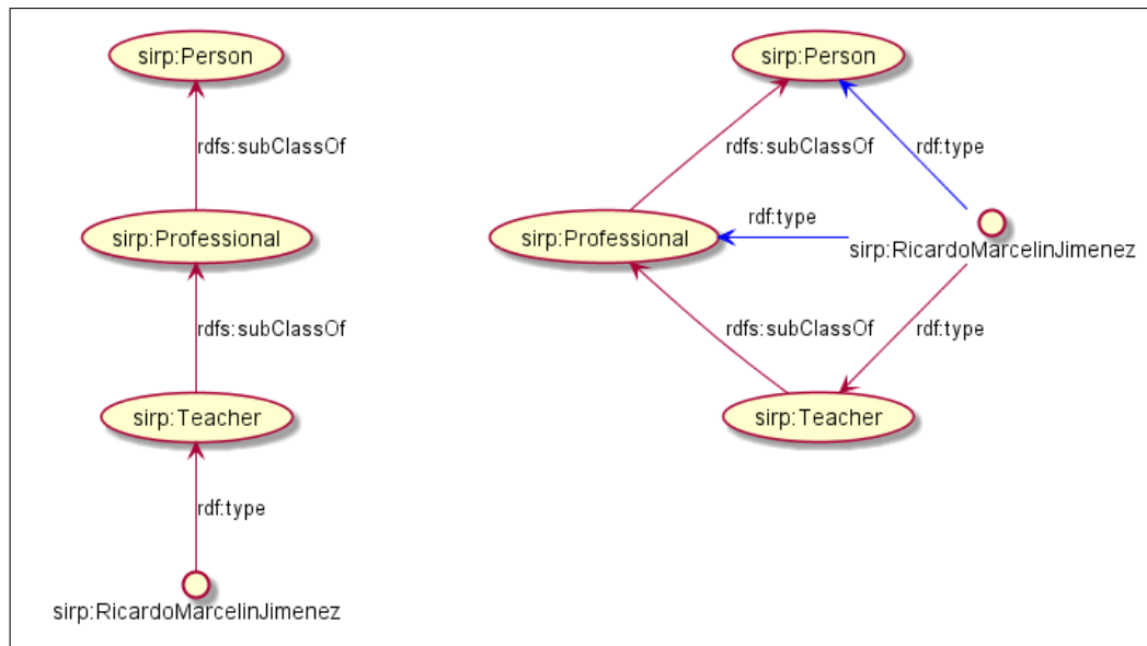
Figura 4.9: Ejemplo de inferencia a partir de los axiomas de jerarquía de clases y el recurso Ricardo Marcelín.
