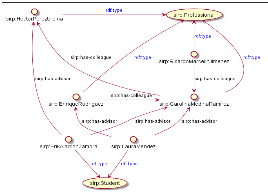
Figura 4.20: Ejemplo de inferencia para los axiomas de dominio y rango que pertenecen a la cartografía de competencias.
