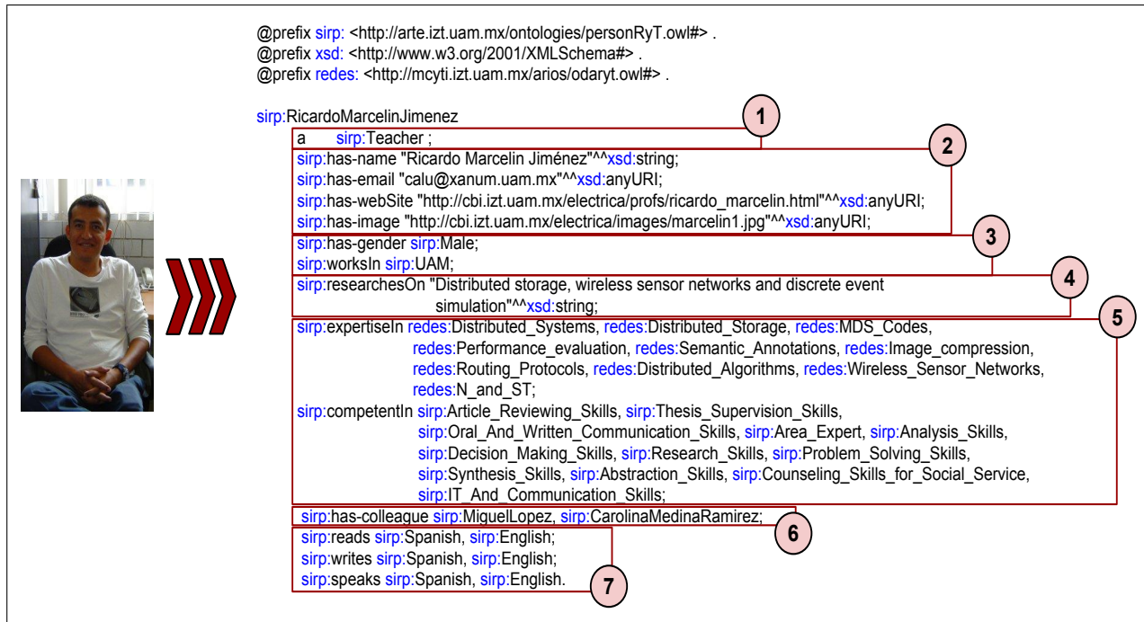
Figura 4.5: Declaraciones del Dr. Ricardo Marcelín Jiménez en forma de tripletas RDF
