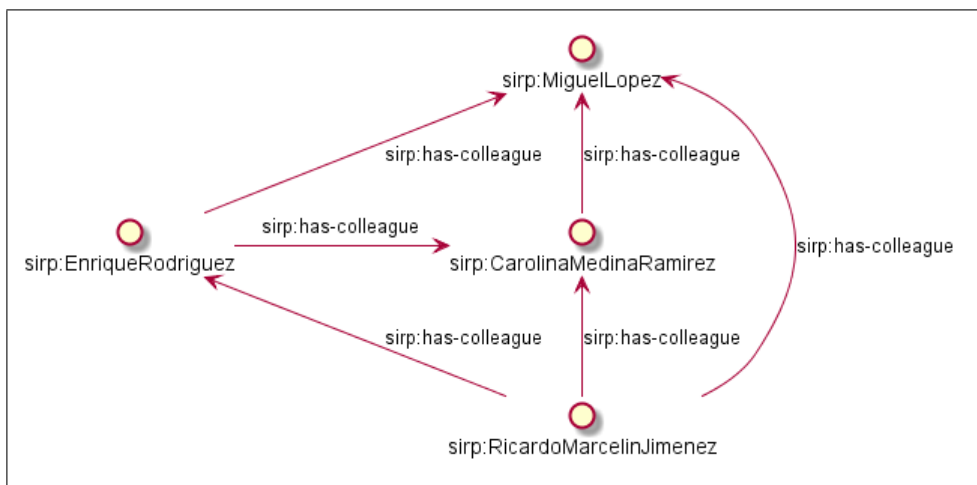
Figura 4.23: Subgrafo RDF con tripletas que indican las relaciones profesionales entre profesores del área.
