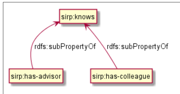
Figura 4.14: Jerarquía de propiedades para las relaciones profesionales entre personas.
