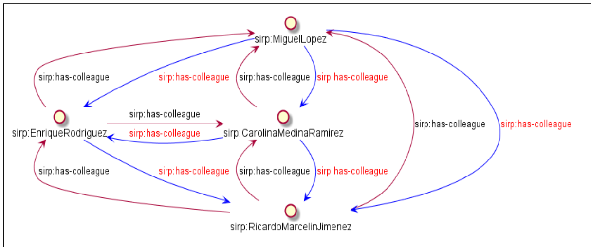
Figura 4.24: Ejemplo de inferencia a partir de la propiedad tiene-colega como propiedad simétrica.
