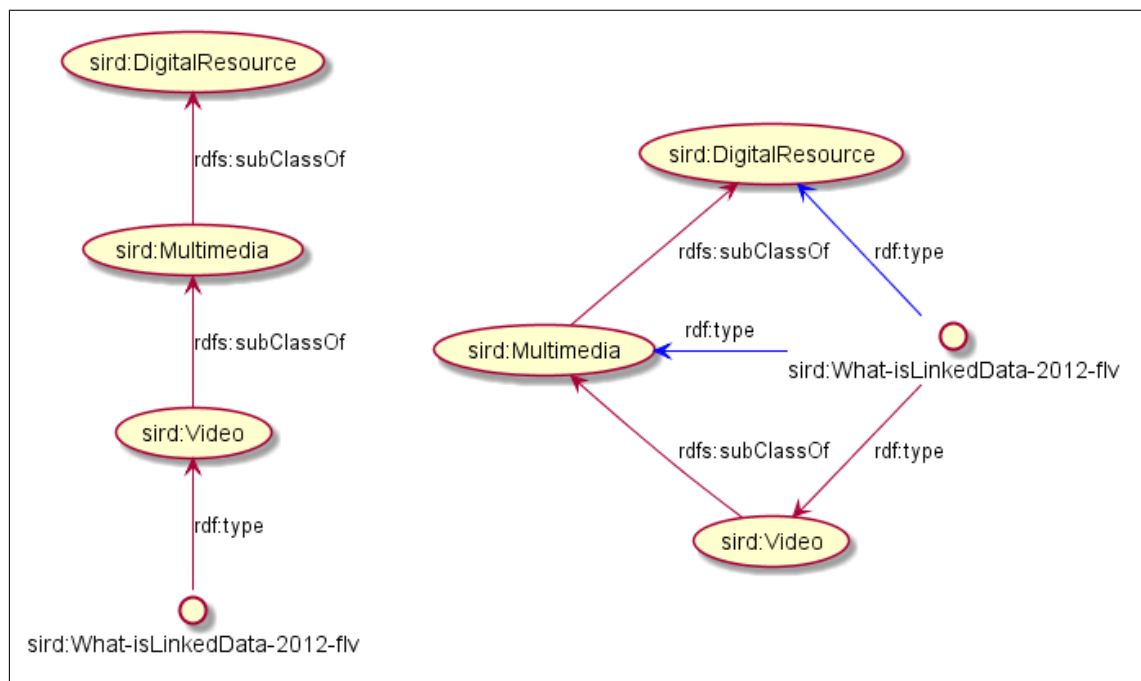
Figura 4.11: Ejemplo de inferencia para los axiomas de jerarquía de clases y el uso del recurso What is Linked Data?
