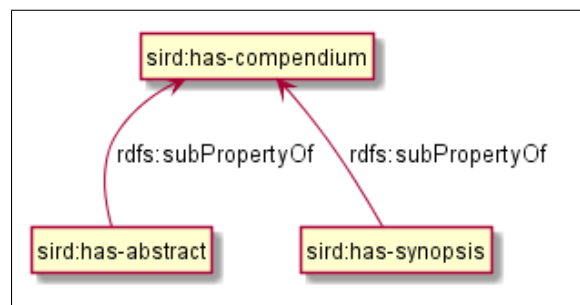
Figura 4.15: Jerarquía de propiedades para describir el contenido de un recurso digital.
