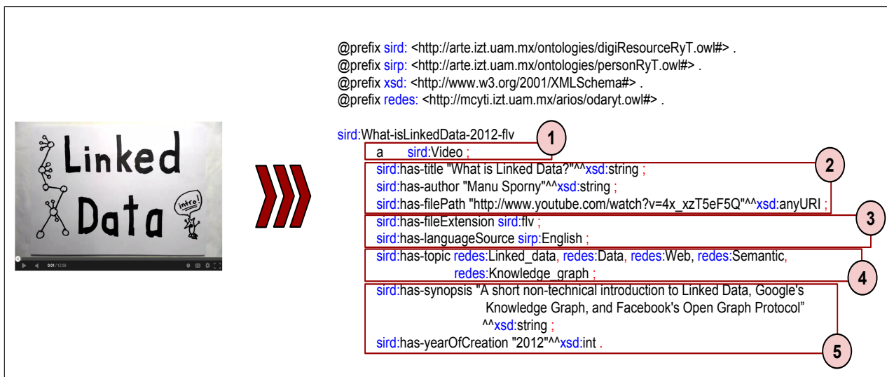
Figura 4.6: Declaraciones de vídeo “What is Linked Data?” en forma de triplas RDF
