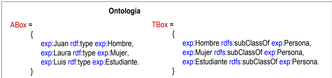
Figura 2.5: ABox y TBox para ejemplificar el beneficio de utilizar un razonador y un motor de búsqueda.
