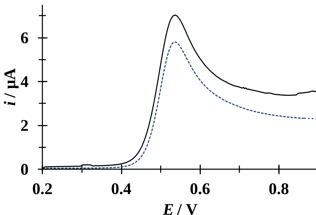
Figura 6.57. VLs experimentales típicas obtenida en el sistema EPC / ACT 64.9 \mu\text{M} , (buffer de fosfatos 0.1M, pH 7) iniciando el barrido de potencial en 0.2 V a una velocidad de 100 \text{ mVs}^{-1} . En línea punteada el VL de ACT en ausencia de CTAB y en línea continua ACT en presencia de CTAB 0.1 mM.
