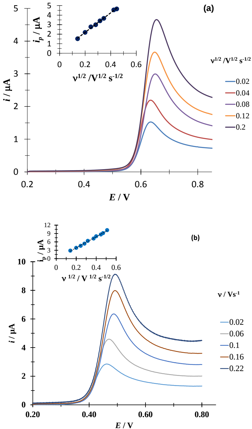
Figura 3.58. VLs experimentales típicas obtenida en el sistema EPC vs Ag/AgCl / ACT 64.9 \mu M en presencia de CTAB 0.1mM, (buffer de fosfatos 0.1M, pH 7) al variar el potencial del electrodo en dirección anódica, iniciando a 0.4 V a diferentes velocidades de barrido del potencial indicadas en la figura. (a) ACT en ausencia de CTAB. (b) ACT en presencia de CTAB 0.1 mM. En los insertos de las figuras se muestra la variación de la corriente de pico anódica ( i_{pa} ) en función de la raíz cuadrada de la velocidad de barrido del potencial ( v ). La línea punteada es la regresión lineal de los datos experimentales (puntos).
