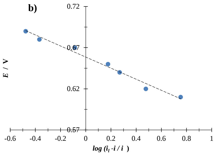
Figura 6.44 (a) Curvas i = f(E) obtenidas a partir de la Figura 6.3 utilizando diferentes tiempos de muestreo indicados en la figura. (b) Curva E = f(\log(i_l - i / i)) para un tiempo de muestreo de 95 ms.
