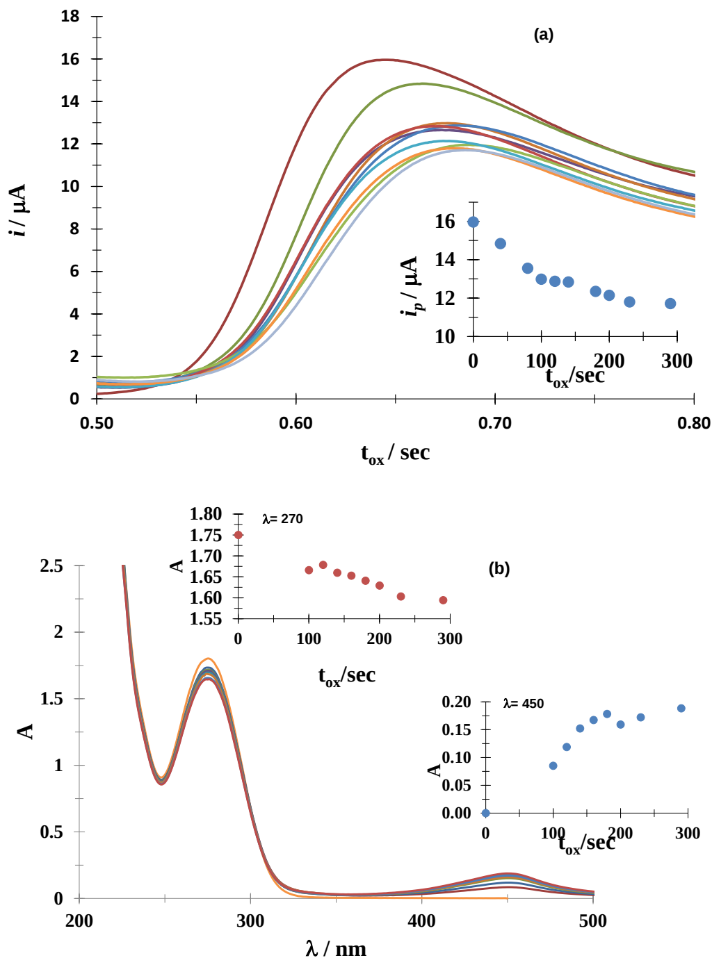
Figura 6.48. Familia de a) VLs, a una velocidad de potencial de 100 \text{ mV s}^{-1} en el sistema malla de Pt/ DCF 209 \mu\text{M} , (PBS 0.1 \text{ M} , pH 7) después de diferentes tiempos de oxidación a 640 \text{ mV} . La dependencia de los picos de corriente de los voltamperogramas y la absorbancia a 270 y 450 \text{ nm} de los espectros UV-vis con el tiempo de oxidación son también representados en los insertos de las figuras a y b respectivamente.
