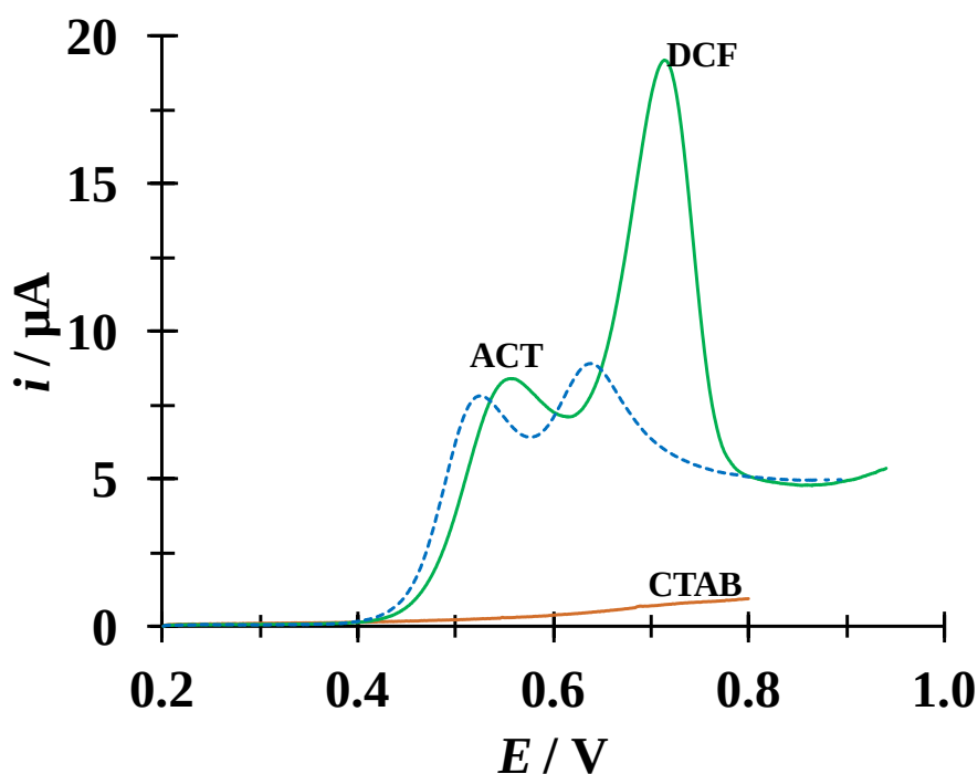
Figura 6.61. VLs experimentales típicas obtenida en el sistema EPC / ACT/DCF (buffer de fosfatos 0.1\text{M} , \text{pH } 7 ) con una concentración de DCF de 51.98 \mu\text{M} y de ACT 51.98 \mu\text{M} . Iniciando el barrido de potencial en 0.2 \text{ V} a una velocidad de 100 \text{ mVs}^{-1} . La línea punteada es DCF en presencia de ACT en ausencia de CTAB, la línea continua es DCF en presencia de ACT en presencia de CTAB.
