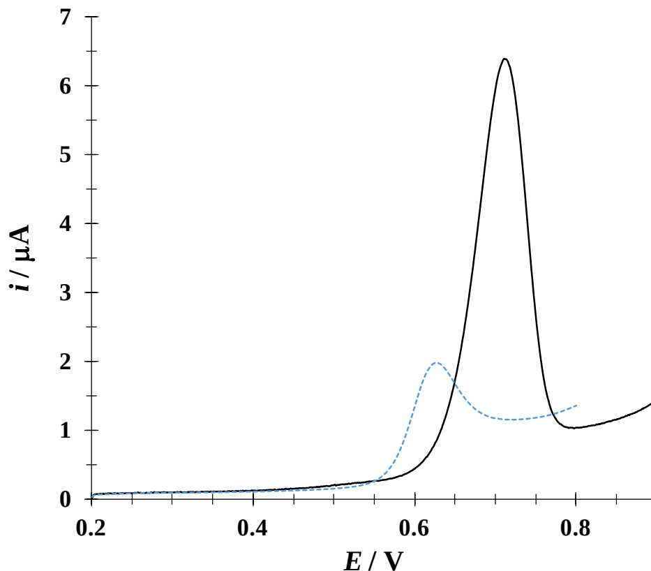
Figura 6.54. VLs experimentales típicas obtenida en el sistema EPC vs Ag/AgCl / DCF 16.34 \mu\text{M} , (buffer de fosfatos 0.1M, pH 7) iniciando el barrido de potencial en 0.2 V a una velocidad de 100 \text{mVs}^{-1} . En línea punteada el VL de DCF en ausencia de CTAB y en línea continua DCF en presencia de CTAB 0.1 mM.
