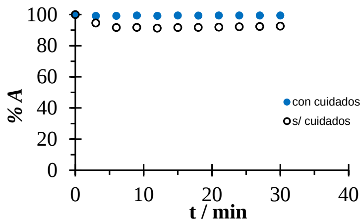
Figura 6.13. % de Absorbancia en función del tiempo para la especie \text{DCF}^- en \text{NaCl} 0.1 M pH 7.
