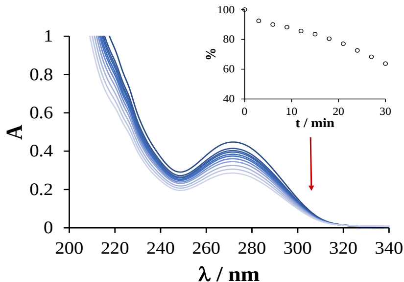
Figura 6.6. Espectros de absorción de DCF 0.5 mM a diferentes tiempos a pH 1.5 en \text{HClO}_4 0.1M.
