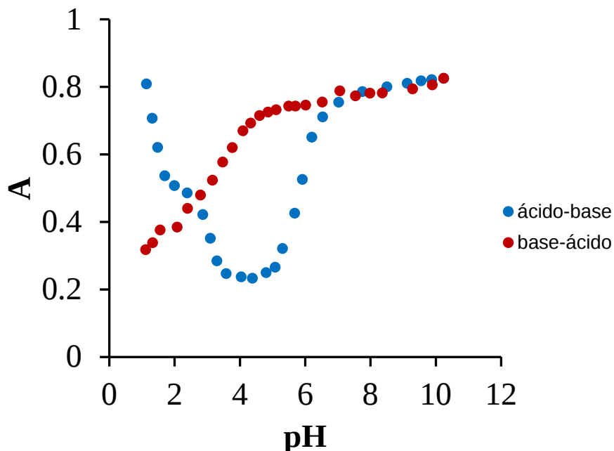
Figura 6.27. Historial de Absorbancias de DCF 0.1mM a 273 nm en cloruros 0.1M comenzando con especie protonada de DCF a diferentes valores de pH.
