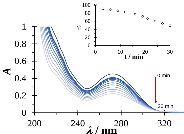
Figura 6.3. Espectros de absorción de DCF 0.5 mM a diferentes tiempos a pH 1.5 en HCl 0.1M.
