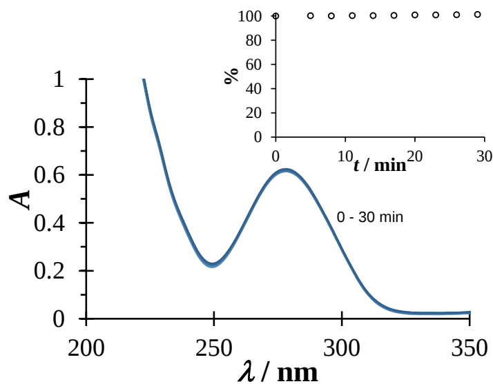
Figura 6.12. Espectros de absorción de DCF 0.5 mM a diferentes tiempos a pH 7 en NaCl 0.1M.
