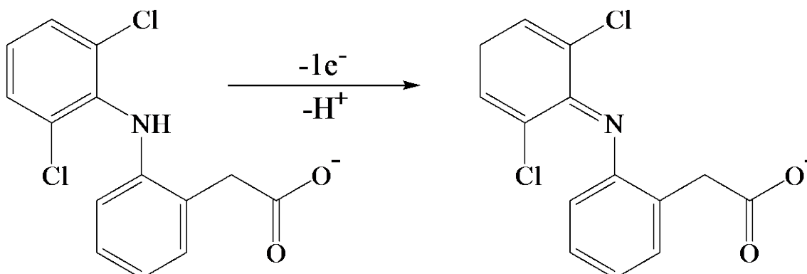
Figura 6.45. Etapa inicial del mecanismo de la oxidación electroquímica del diclofenaco en disolución acuosa a pH 7 utilizando un electrodo de pasta de carbono.
