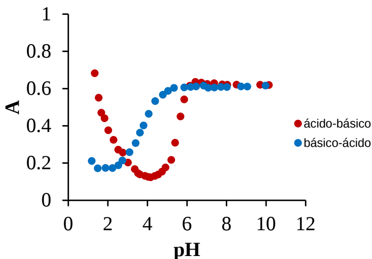
Figura 6.35. Historial de Absorbancias de DCF 0.1mM a 273 nm en fosfatos 0.1M comenzando con especie protonada de DCF a diferentes valores de pH.
