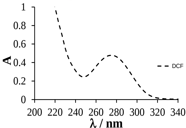
Figura 6.14. Espectro de absorción de DCF 0.5 mM pH 7 en \text{NaClO}_4 0.1 M
