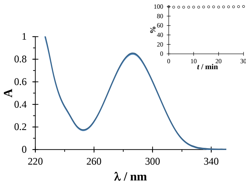
Figura 6.21. Espectros de absorción de DCF 0.5 mM a diferentes tiempos a pH 7 en HCl 0.1M en presencia de CTAB 0.6mM.
