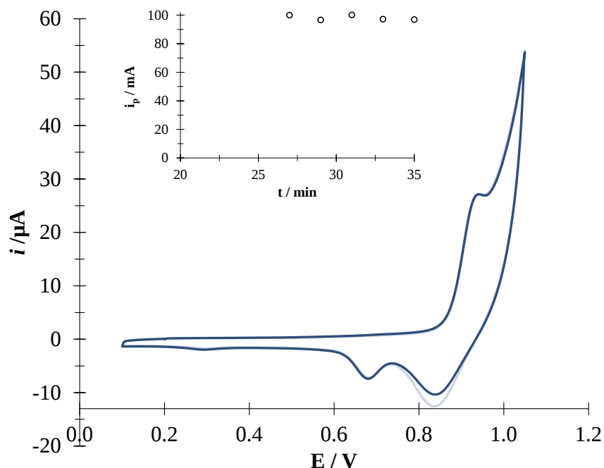
Figura 6.24 .VC de la especie DCFH en presencia de CTAB 0.6 mM en HCl 0.1 M, EPC vs Ag/AgCl a 0.1 \text{ V s}^{-1}
