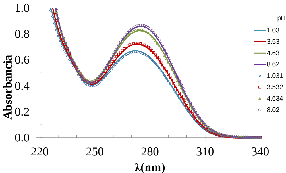
Figura 6.38. Espectros UV-Vis de DCF 0.1 mM en fosfatos 0.1 M ajustados a partir de los datos calculados (línea) y comparados con los experimentales (marcador).
