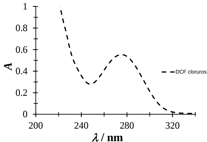
Figura 6.11 .Espectro de absorción de DCF 0.5 mM en NaCl 0.1 M pH 7.
