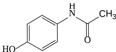
Figura 2.5. Estructura molecular de acetaminofén.
