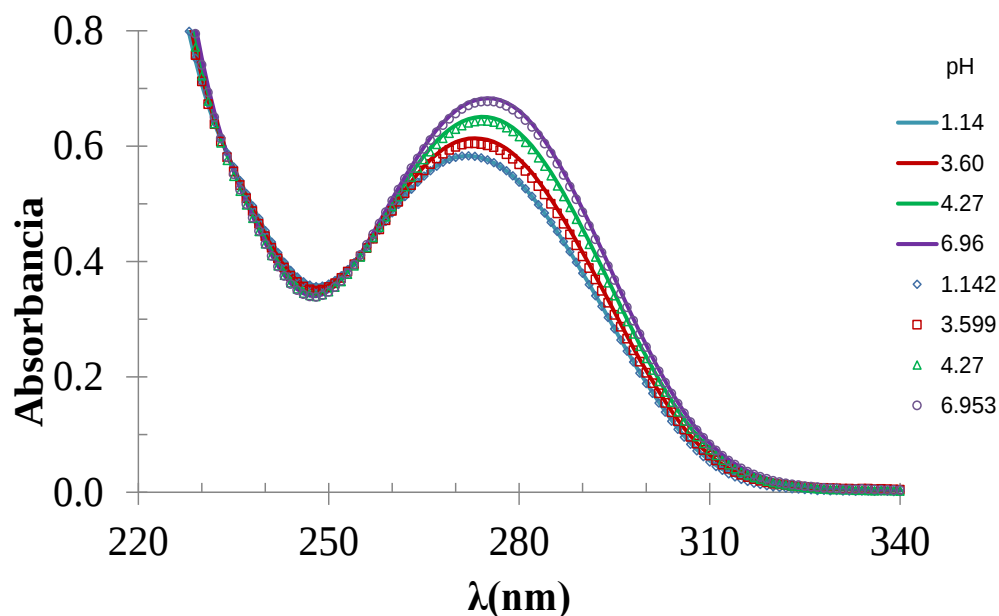
Figura 6.34. Espectros UV-Vis de DCF 0.1 mM en percloratos ajustados a partir de los datos calculados (línea) y comparados con los experimentales (marcador).
