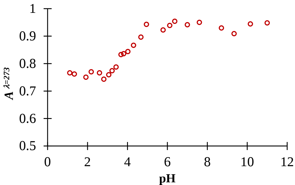
Figura 6.28. Historial de Absorbancias de DCF 0.1mM a 273 nm en cloruros 0.1M comenzando con especie aniónica de DCF a diferentes valores de pH.
