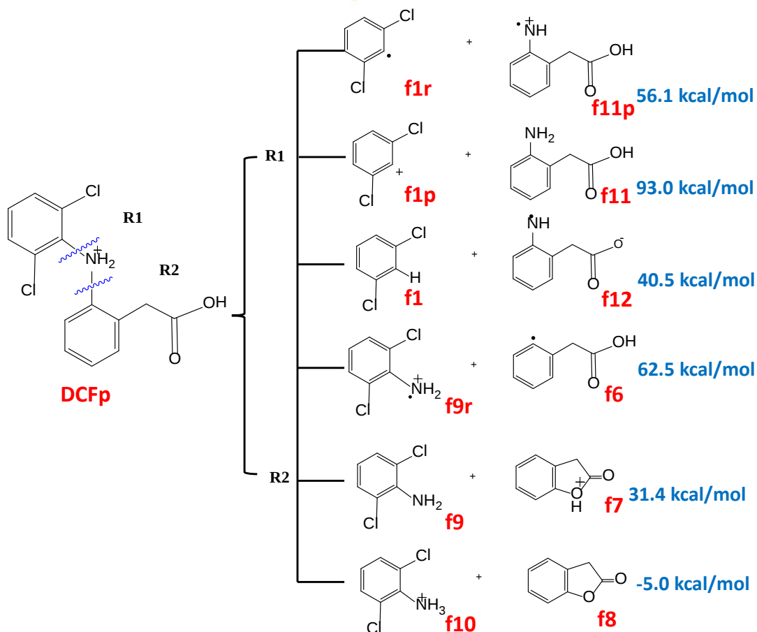
Esquema II. Rutas de descomposición de DCF propuestas partiendo de molécula protonada.
