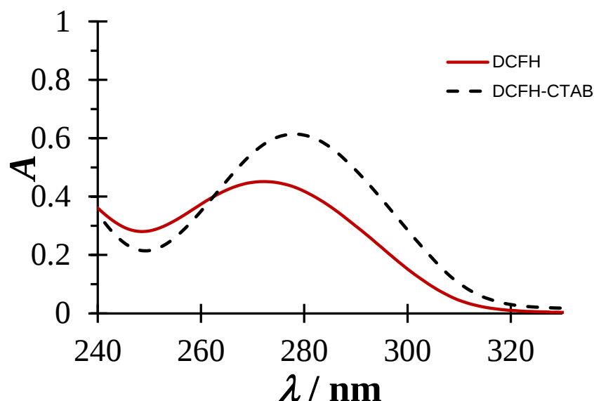
Figura 6.20. Espectros de absorción de la especie DCFH en presencia y ausencia de CTAB 0.6 mM en HCl 0.1M pH 1.5.
