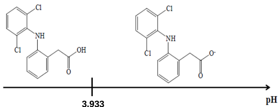
Figura 6.41. Diagrama de Zona de predominio Lineal de DCF.
