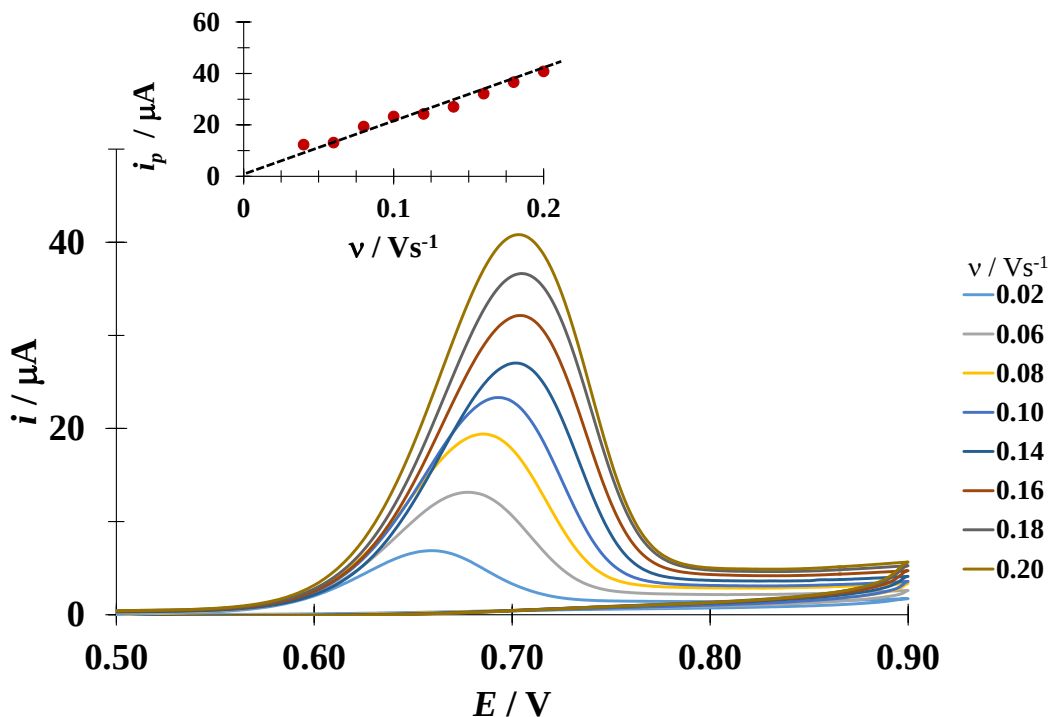
Figura 6.55. VLs experimentales típicas obtenida en el sistema EPC vs Ag/AgCl / DCF 100.0μM en presencia de CTAB 0.1mM, (buffer de fosfatos 0.1M, pH 7) al variar el potencial del electrodo en dirección anódica, iniciando a 0.4 V) a diferentes velocidades de barrido del potencial indicadas en la figura. El inserto muestra la variación de la corriente de pico anódica ( i_{pa} ) en función de la velocidad de barrido del potencial ( \nu ). La línea punteada es la regresión lineal de los datos experimentales (puntos).
