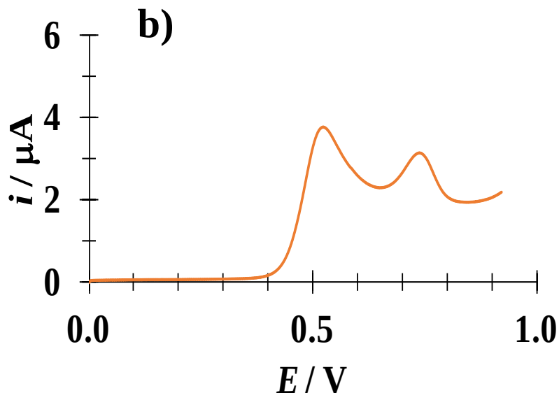
Figura 6.64. VLs experimentales obtenidos en el sistema EPC / Ag/AgCl (buffer de fosfatos 0.1M, pH 7). Iniciando el barrido de potencial en 0.0 V a una velocidad de 100 mVs^{-1} . En (a) en ausencia de CTAB y en (b) en presencia de CTAB 40 \mu M .
