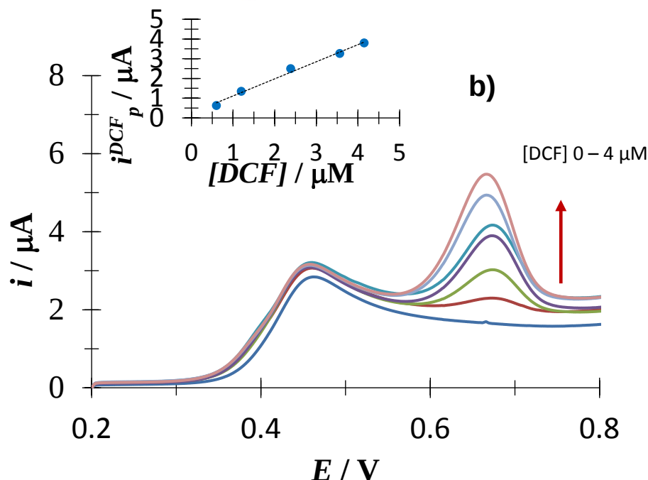
Figura 6.62. VLs experimentales típicas obtenida en el sistema EPC / ACT/ DCF (buffer de fosfatos 0.1M, pH 7) para una concentración fija de ACT de 48.8 \mu M . Iniciando el barrido de potencial en 0.2 V a una velocidad de 100 mVs^{-1} para diferentes concentraciones de DCF, indicadas en la figura. En (a) en ausencia de CTAB 0.1mM y en (b) en presencia de CTAB 0.1mM. El inserto de las figuras se muestra la variación de la corriente de pico anódica ( i_p ) en función de la concentración de DCF. La línea punteada es la regresión lineal de los datos experimentales (puntos).
