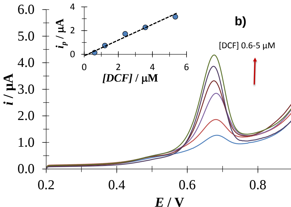
Figura 6.59. VLs experimentales típicas obtenida en el sistema EPC / DCF (buffer de fosfatos 0.1M, pH 7) iniciando el barrido de potencial en 0.2 V a una velocidad de 100 \text{ mVs}^{-1} para diferentes concentraciones de DCF, indicadas en la figura. En (a) DCF en ausencia de CTAB 0.1mM y en (b) DCF en presencia de CTAB 0.1mM. El inserto de las figuras se muestra la variación de la corriente de pico anódica ( i_p ) en función de la concentración de DCF. La línea punteada es la regresión lineal de los datos experimentales (puntos).
