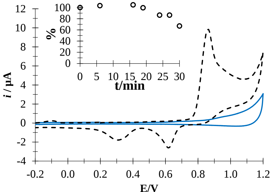
Figura 6.10. VC de la especie DCFH en HCl 0.1 M pH 1.5, EPC vs Ag/AgCl a 0.1 \text{ V s}^{-1}
