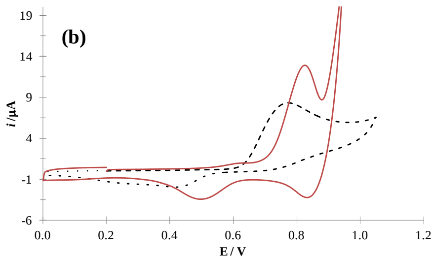
Figura 6.26. Comparación de VC's a 0.1\text{Vs}^{-1} sobre un EPC vs AgCl/Cl de: (a) DCF 1 mM, pH 1 y CTAB 0.6 mM (línea continua), ausencia CTAB (línea punteada) en HCl 0.1 M. (b) DCF 1 mM, pH 7 y CTAB 0.6 mM (línea continua), ausencia CTAB (línea punteada) en NaCl 0.1 M.
