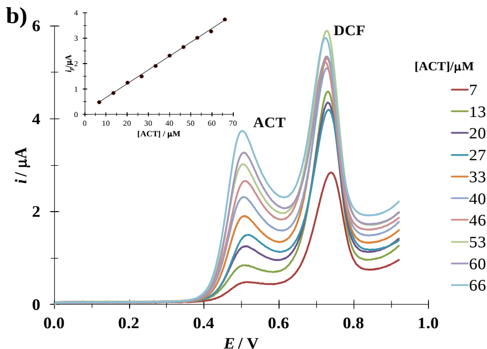
Figura 6.63. VLs experimentales típicas obtenida en el sistema EPC / ACT/ DCF (buffer de fosfatos 0.1M, pH 7) para una concentración fija de DCF de 6.5 \mu\text{M} . Iniciando el barrido de potencial en 0.0 V a una velocidad de 100 \text{ mVs}^{-1} para diferentes concentraciones de ACT, indicadas en la figura. En (a) en ausencia de CTAB y en (b) en presencia de CTAB 40 \mu\text{M} . El inserto de las figuras se muestra la variación de la corriente de pico anódica ( i_p ) en función de la concentración de ACT. La línea punteada es la regresión lineal de los datos experimentales (puntos).
