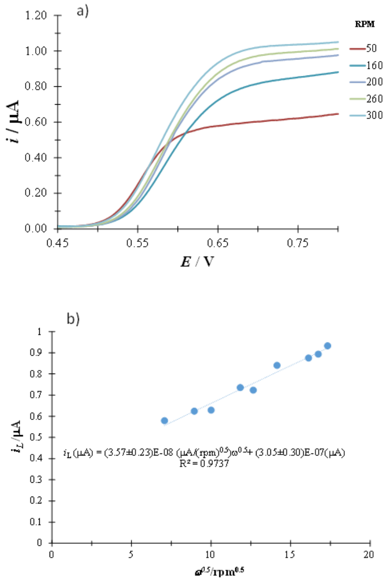
Figura 6.50. a) LVs experimentales típicos obtenidos en el sistema EPC/ DCF 31.1 \mu\text{M} , (PBS 0.1 \text{ M} , pH 7) la velocidad de barrido de potencia comienza en 0.3 \text{ V} a 10 \text{ mV s}^{-1} y aplicando diferentes velocidades de rotación del electrodo, indicado en la figura. b) Variación de la corriente límite anódica como una función de la raíz cuadrada de la velocidad de rotación del electrodo. La línea corresponde a la regresión lineal y los marcadores a los datos experimentales. De la pendiente de la ecuación, y de la ecuación de Levich (2.4) el valor del coeficiente de difusión de DCF fue determinado (7.82 \pm 0.63) \times 10^{-6} \text{ cm}^2\text{s}^{-1} .
