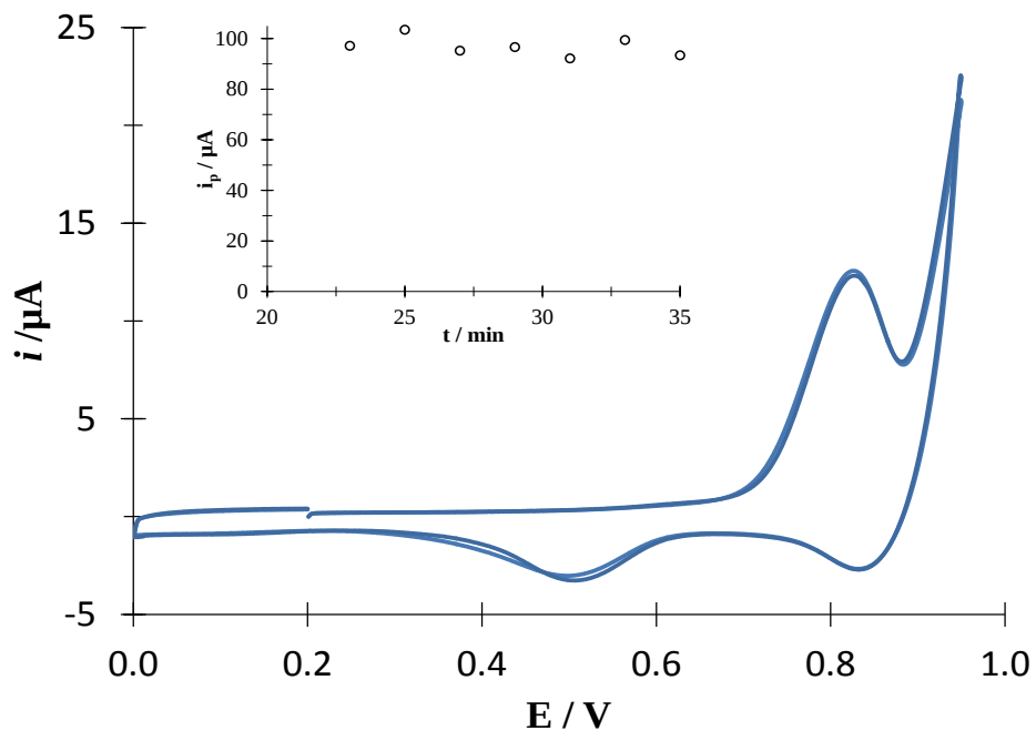
Figura 6.25 .VC de la especie \text{DCF}^- en presencia de CTAB 0.6 mM en NaCl 0.1 M, EPC vs Ag/AgCl a 0.1 \text{ V s}^{-1}
