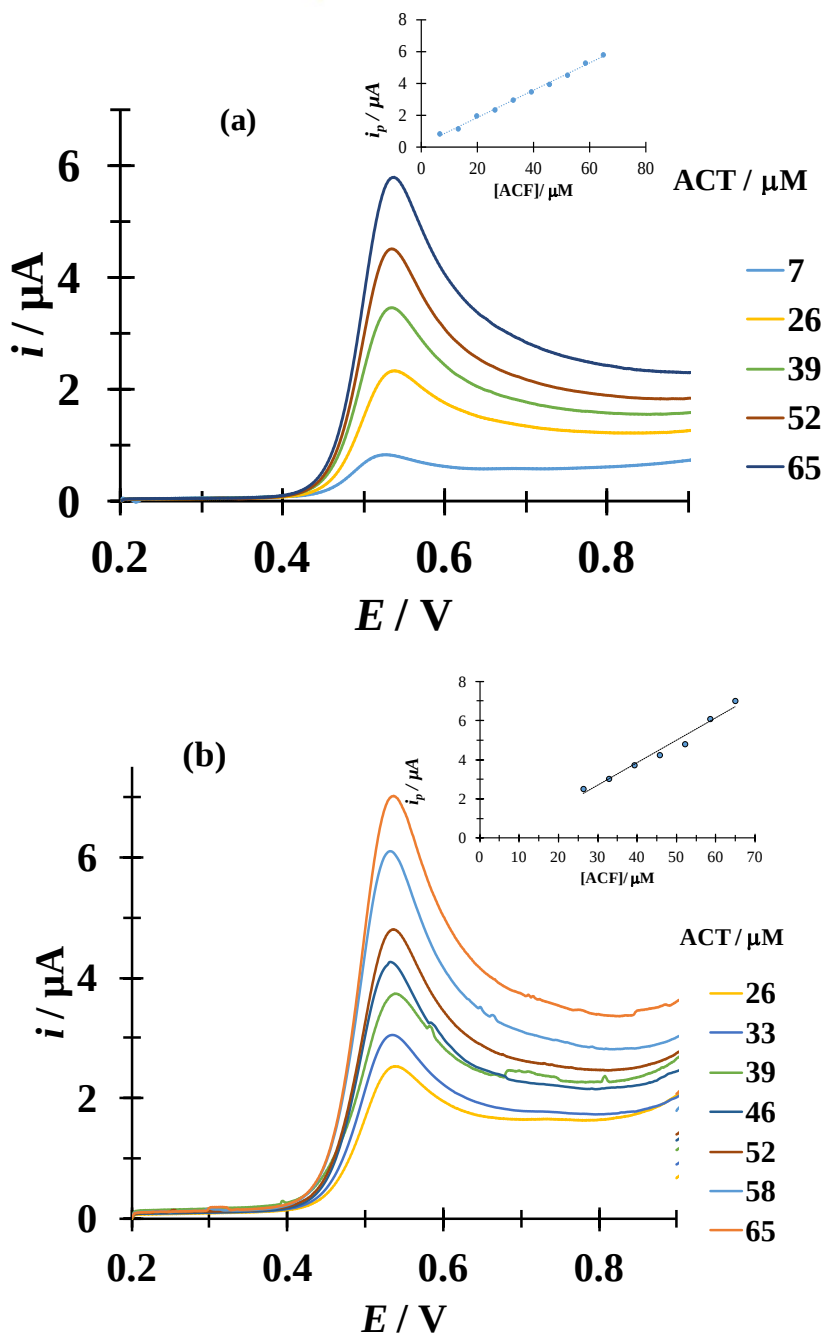
Figura 6.60. VLs experimentales típicas obtenida en el sistema EPC / ACT (buffer de fosfatos 0.1M, pH 7) iniciando el barrido de potencial en 0.2 V a una velocidad de 100 \text{ mVs}^{-1} para diferentes concentraciones de ACT, indicadas en la figura. En (a) ACT en ausencia de CTAB 0.1mM y en (b) ACT en presencia de CTAB 0.1mM. El inserto de las figuras se muestra la variación de la corriente de pico anódica ( i_p ) en función de la concentración de ACT. La línea punteada es la regresión lineal de los datos experimentales (puntos).
