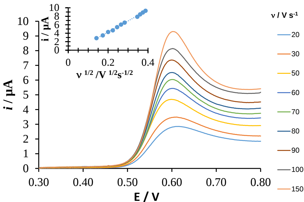
Figura 6.42. VLs experimentales típicas obtenida en el sistema EPC/ DCF 142 \mu\text{M} , (buffer de fosfatos 0.1M, pH 7) al variar el potencial del electrodo en dirección anódica, iniciando a 0.3 V) a diferentes velocidades de barrido del potencial indicadas en la figura. El inserto muestra la variación de la corriente de pico anódica ( i_{pa} ) en función de la raíz cuadrada de la velocidad de barrido del potencial ( \nu ). La línea punteada es la regresión lineal de los datos experimentales (puntos).
