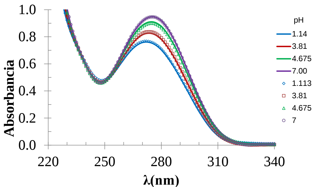
Figura 6.30. Espectros UV-Vis de DCF 0.1 mM en cloruros ajustados a partir de los datos calculados (línea) y comparados con los experimentales (marcador).
