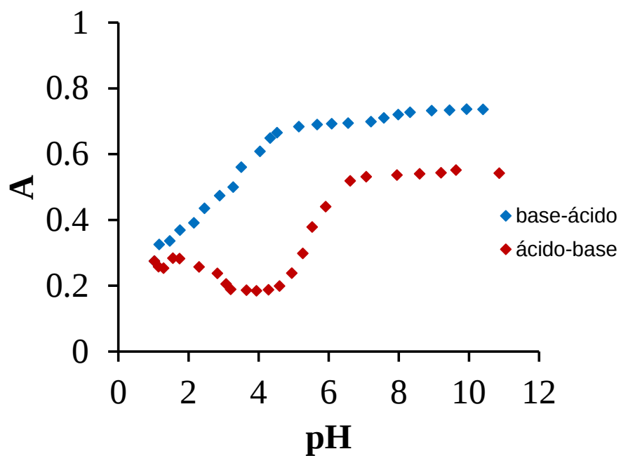
Figura 6.28. Historial de Absorbancias de DCF 0.1mM a 273 nm en cloruros 0.1M comenzando con especie aniónica de DCF a diferentes valores de pH.
