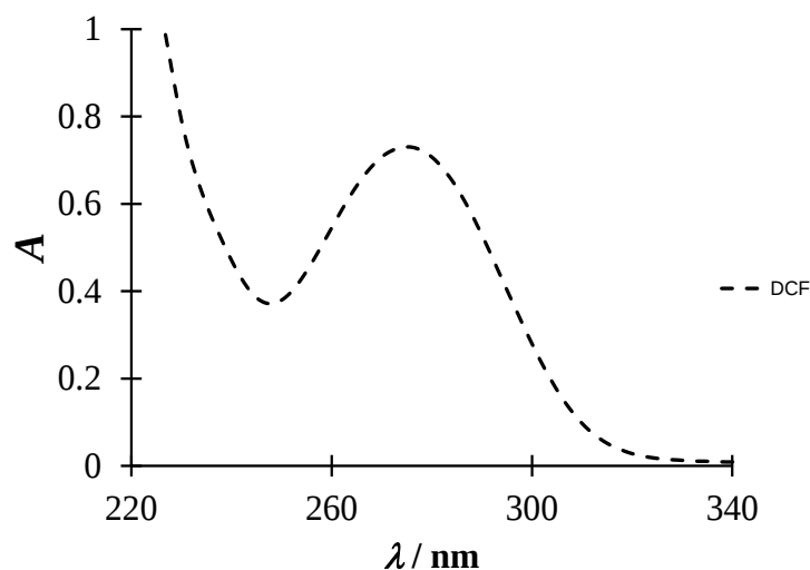
Figura 6.16. Espectro de absorción de DCF 0.5 mM a pH 7 en fosfatos 0.1 M.
