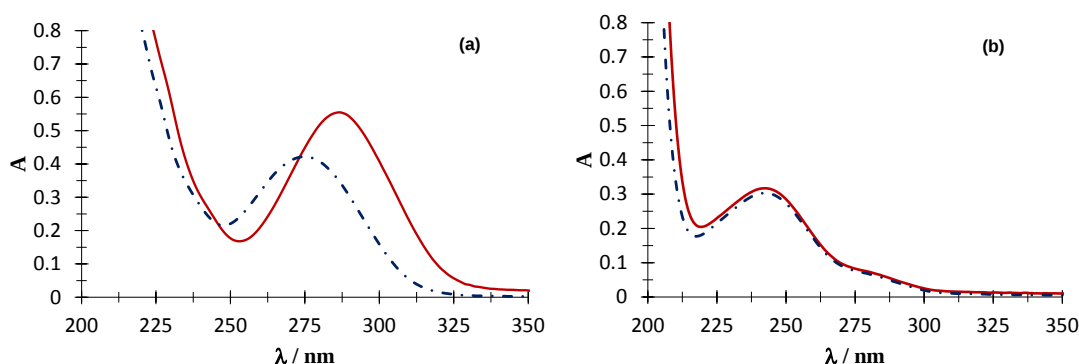
Figura 6.52. Espectros de absorción de UV-Vis para el sistema de buffer fosfatos pH 7 0.1M. En línea continua se presentan los espectros en presencia de CTAB 0.1 mM y en línea punteada en ausencia de CTAB. (a) DCF 64 μM y (b) ACT 64 μM.
