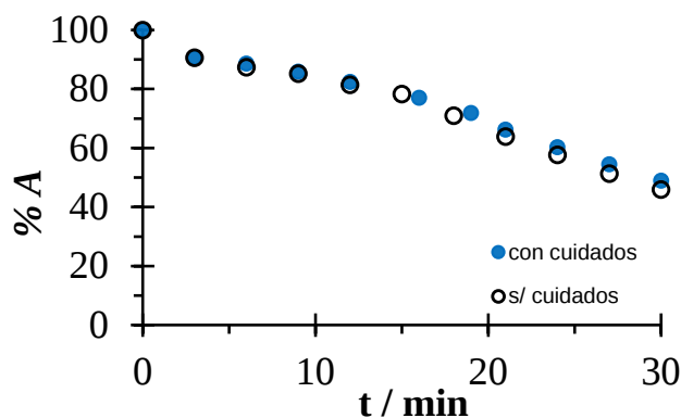
Figura 6.4. % de Absorbancia en función del tiempo para la especie DCFH en HCl 0.1 M
