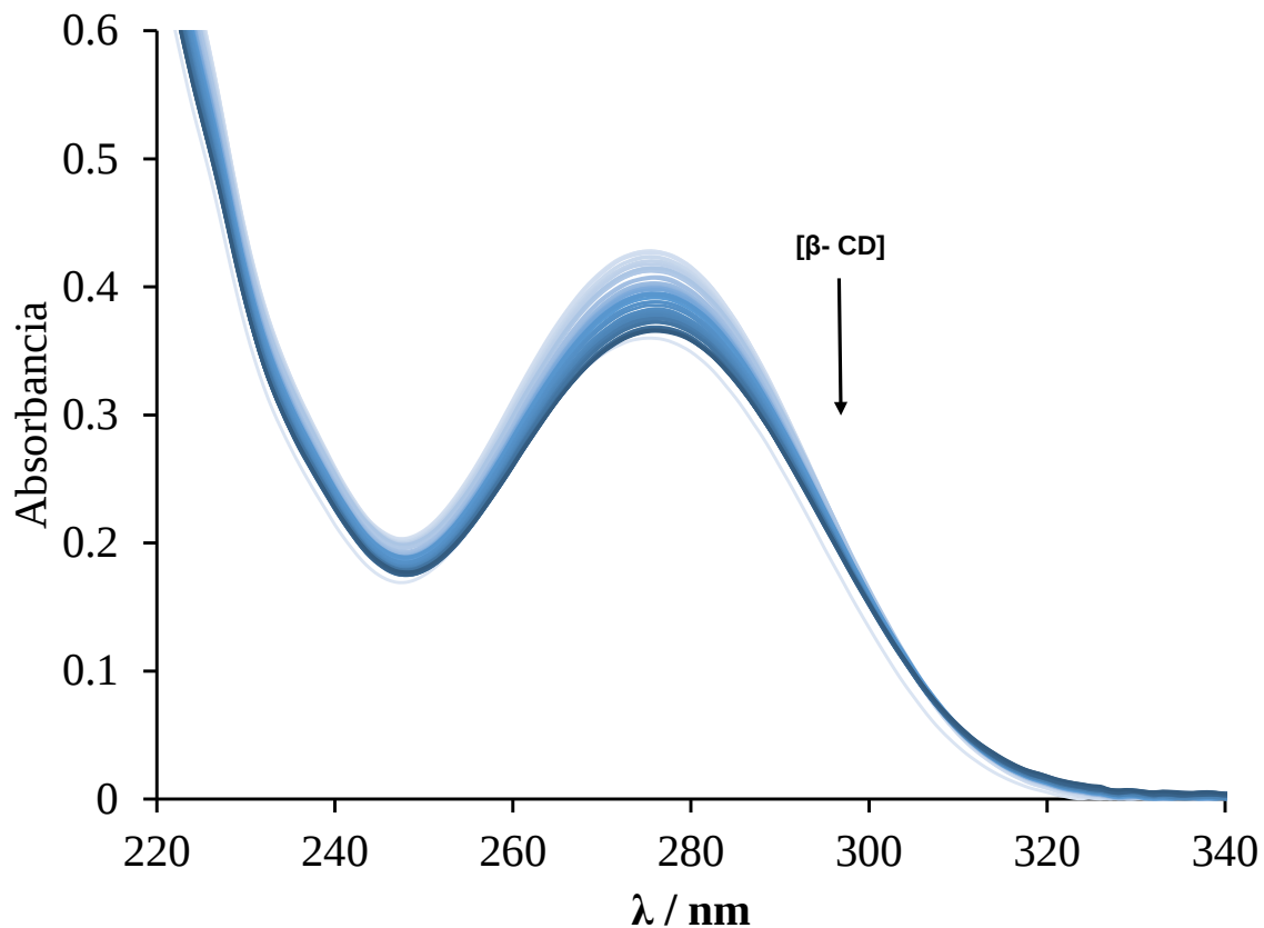
Figura 6.65 .Espectros de absorción obtenidos en una de DCF 32.7 mM a pH 7 y diferentes valores de concentraciones de \beta -CD, indicadas en la figura en mM.
