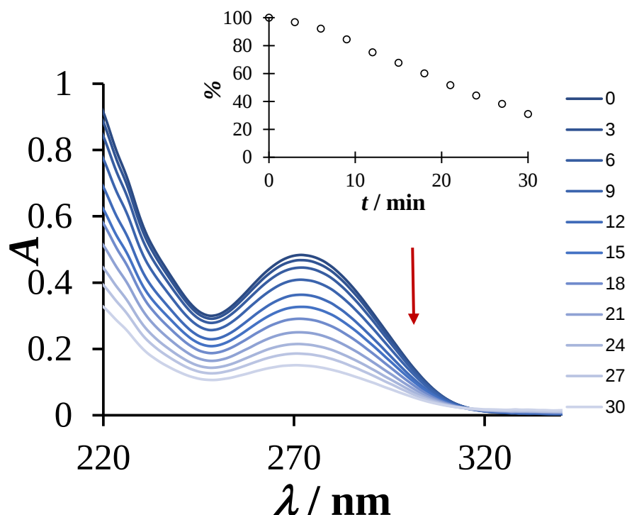
Figura 6.9. Espectros de absorción de DCF 0.5 mM a diferentes tiempos a pH 1.5 en \text{H}_3\text{PO}_4 0.1M.
