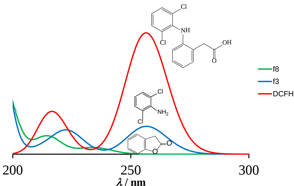
Figura 6.39. Espectros de absorción para la especie neutra (DCFH) y de sus productos de degradación (f8 y f3).
