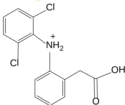
Figura 2.4 .Estructura molecular de diclofenaco protonado.
