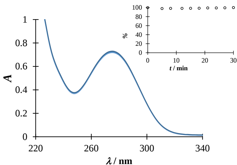
Figura 6.17. Espectros de absorción de DCF 0.5 mM a diferentes tiempos a pH 7 en fosfatos 0.1M.
