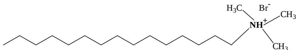
Figura 2.6. Estructura molecular de CTAB.
