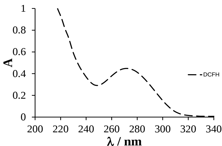
Figura 6.5. .Espectro de absorción de DCF 0.5 mM a pH 1.5 en \text{HClO}_4 0.1M
