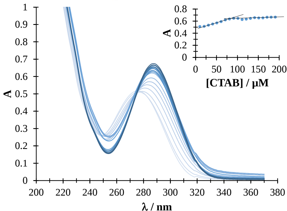
Figura 6.53. Familia de espectros UV-Vis obtenidos en el sistema DCF 0.5 mM, en buffer fosfatos pH 7 0.1 M a para diferentes concentraciones de CTAB mostradas en la figura. En el inserto se presenta la variación de la absorbancia (288 nm) en función de la concentración de CTAB.
