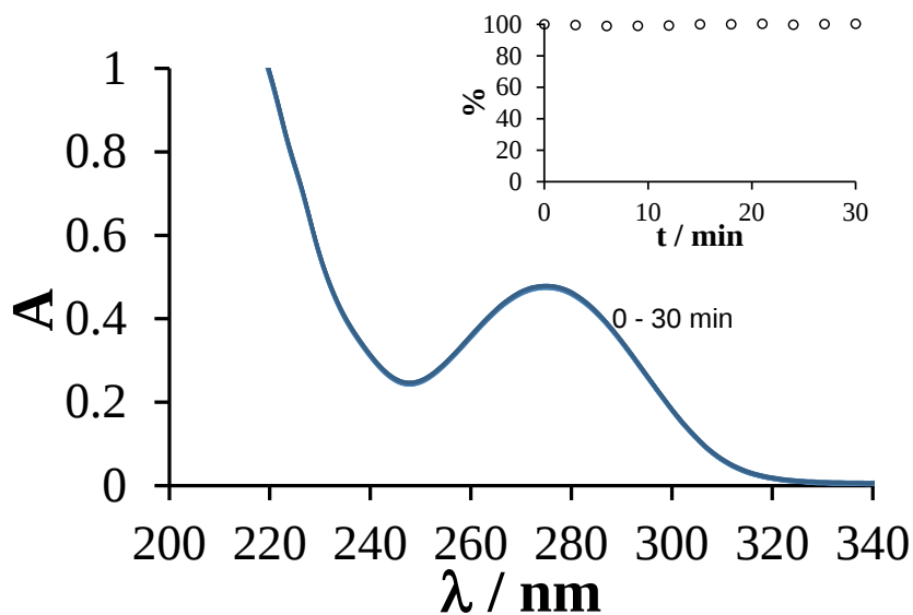
Figura 6.15. Espectros de absorción de DCF 0.5 mM a diferentes tiempos a pH 7 en \text{NaClO}_4 0.1 M.
