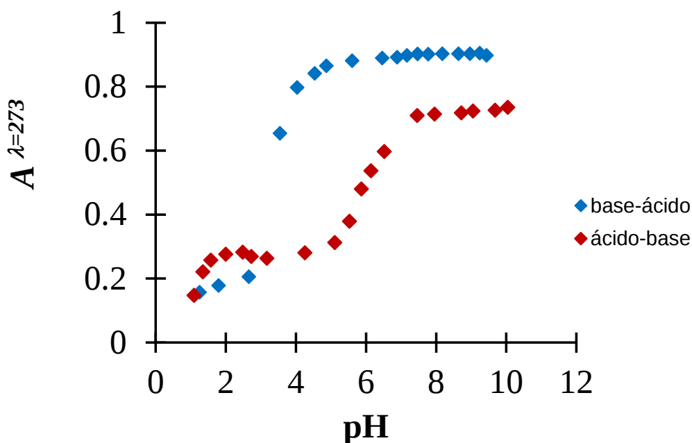
Figura 6.32. Historial de Absorbancias de DCF 0.1mM a 273 nm en percloratos 0.1M comenzando con especie aniónica de DCF a diferentes valores de pH.
