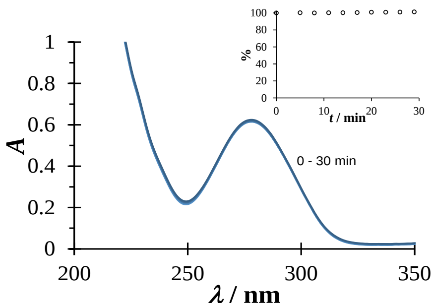
Figura 6.19 Espectros de absorción de DCF 0.5 mM a diferentes tiempos a pH 1.5 en HCl 0.1M en presencia de CTAB 0.6mM.
