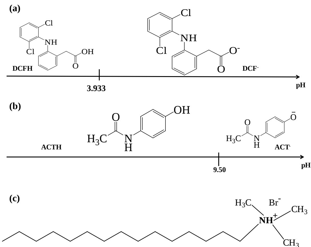
Figura 6.51. Diagrama de Zonas de Predominio Lineal: (a) DCF y (b) ACT construido bajo la metodología propuesta por Rojas-Hernández et al. [32-35]. (c) molécula de Cetiltrimetilamonio.
