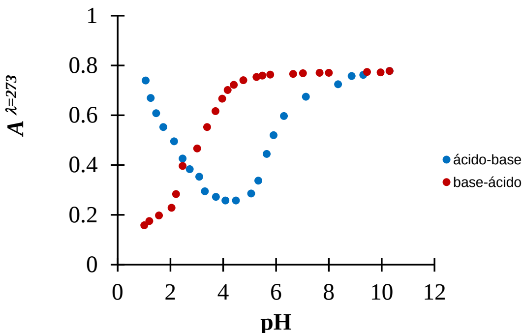
Figura 6.31. Historial de Absorbancias de DCF 0.1mM a 273 nm en percloratos 0.1 M comenzando con especie protonada de DCF a diferentes valores de pH.
