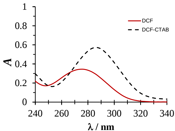
Figura 6.22. Espectros de absorción de la especie \text{DCF}^- en presencia y ausencia de CTAB 0.6 mM en NaCl 0.1M pH 7.
