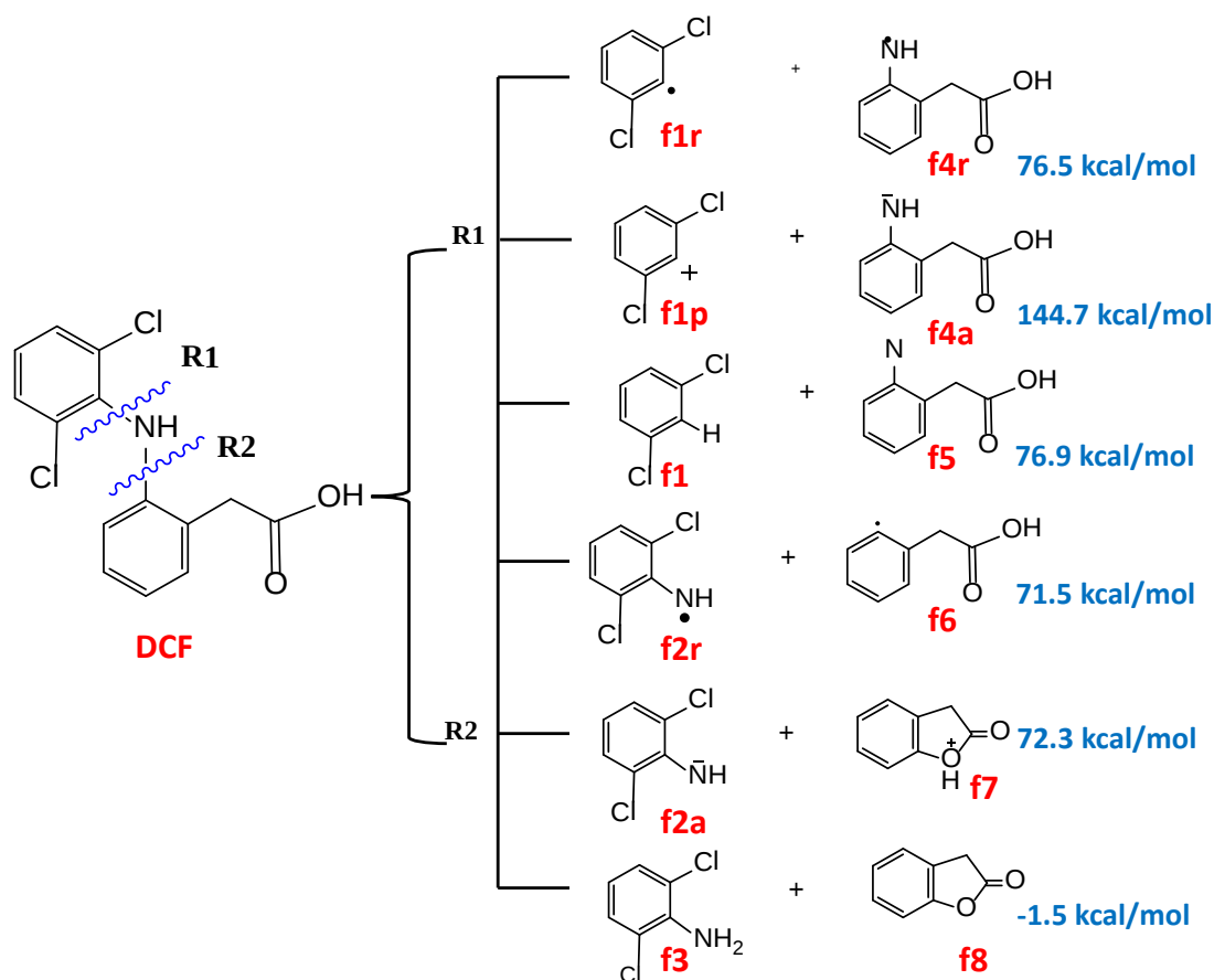
Esquema I. Rutas de descomposición de DCF propuestas partiendo de molécula neutra.
