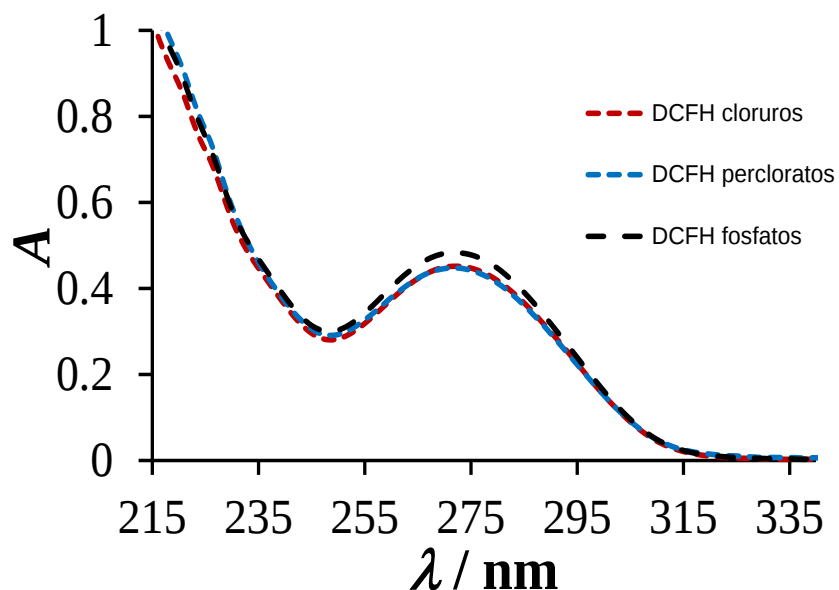
Figura 6.8 .Espectros de absorción de la especie DCFH a pH 1.5 en diferentes iones.
