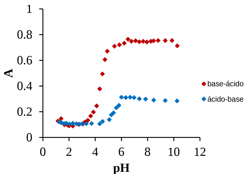
Figura 6.36. Historial de Absorbancias de DCF 0.1mM a 273 nm en fosfatos 0.1M comenzando con especie aniónica de DCF a diferentes valores de pH.
