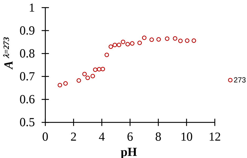
Figura 6.37. Absorbancias a 273 nm para DCF 0.1 mM en fosfatos 0.1M a diferentes valores de pH.
