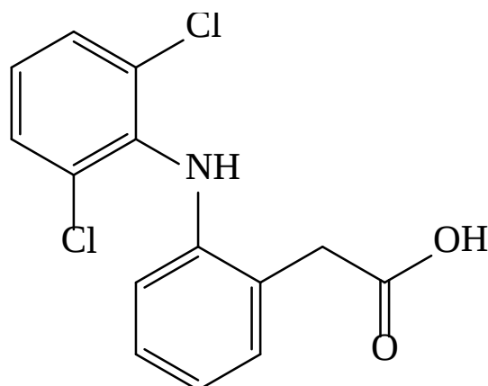
Figura 2.2. Estructura molecular de diclofenaco.
