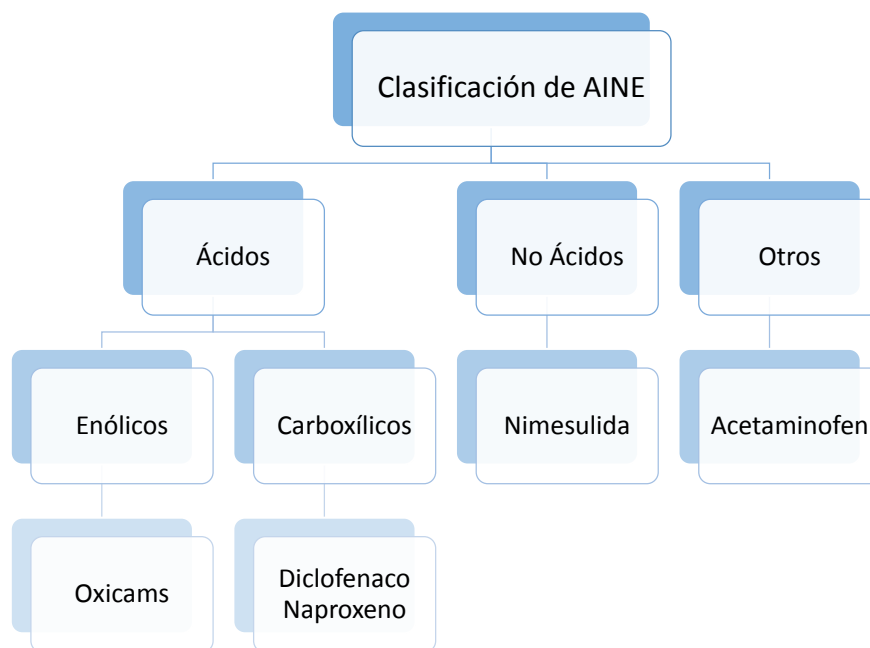
Figura 2.1. Clasificación de antiinflamatorios de acuerdo a su estructura química.
